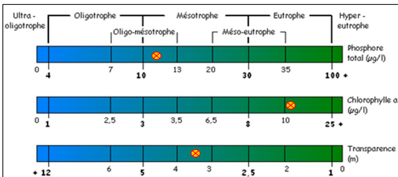
Figure 9 - État trophique 2021 - Lac Lachaine (LA1))
