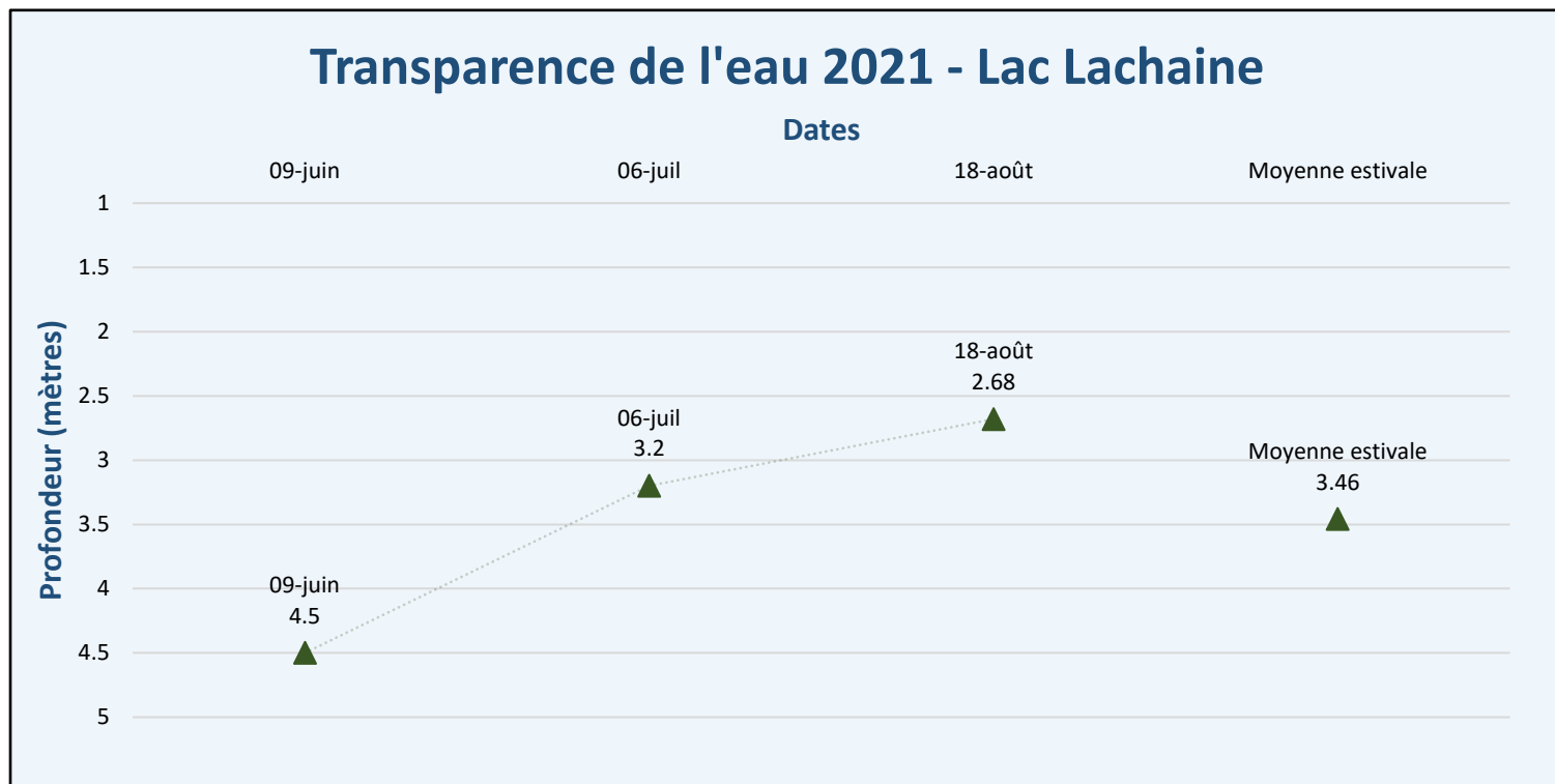
Figure 5 – Résultats transparence de l'eau 2021 – Lac Lachaine
