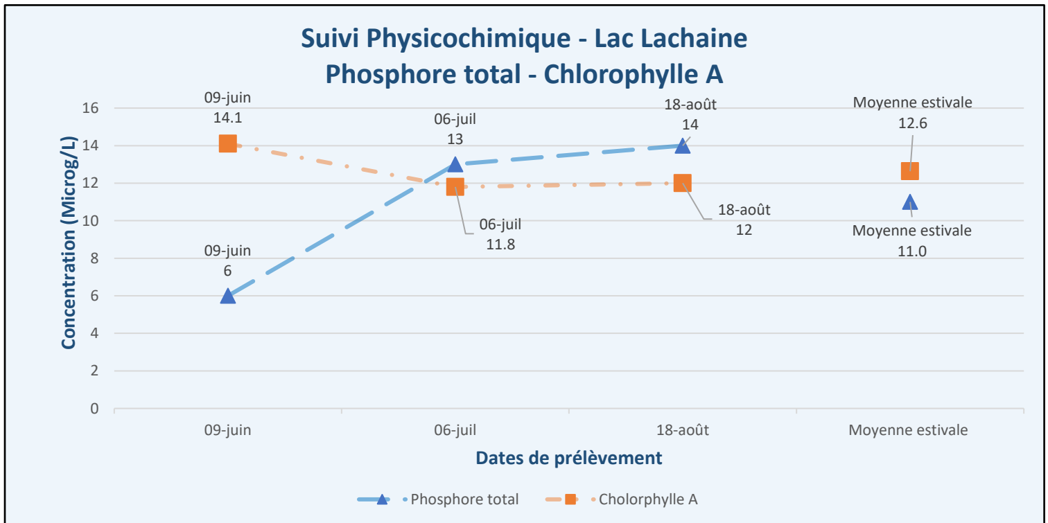
Figure 6 - Résultats – Suivi physicochimique 2021 (PT, Chla) – Lac Lachaine (LA1)
