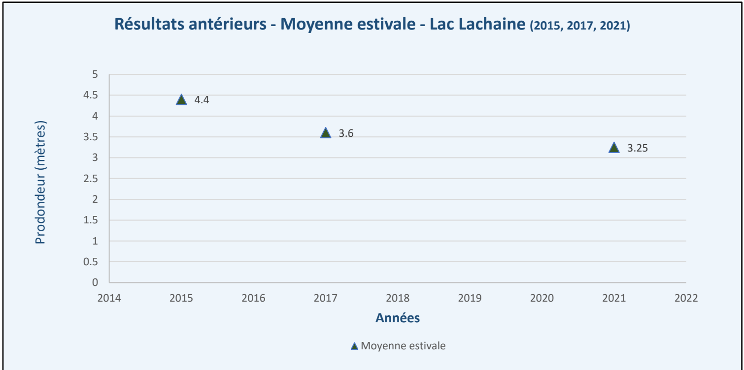
Figure 8 - Résultats antérieurs - Transparence de l'eau – Lac Lachaine (LA1)
