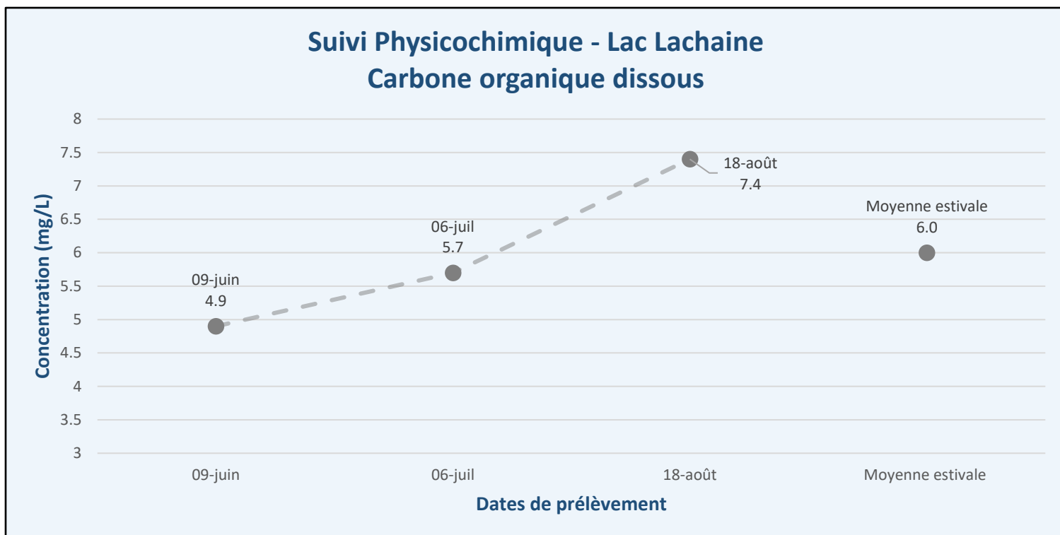
Figure 7 - Résultats – Suivi physicochimique 2021 (COD) - Lac Lachaine (LA1)
