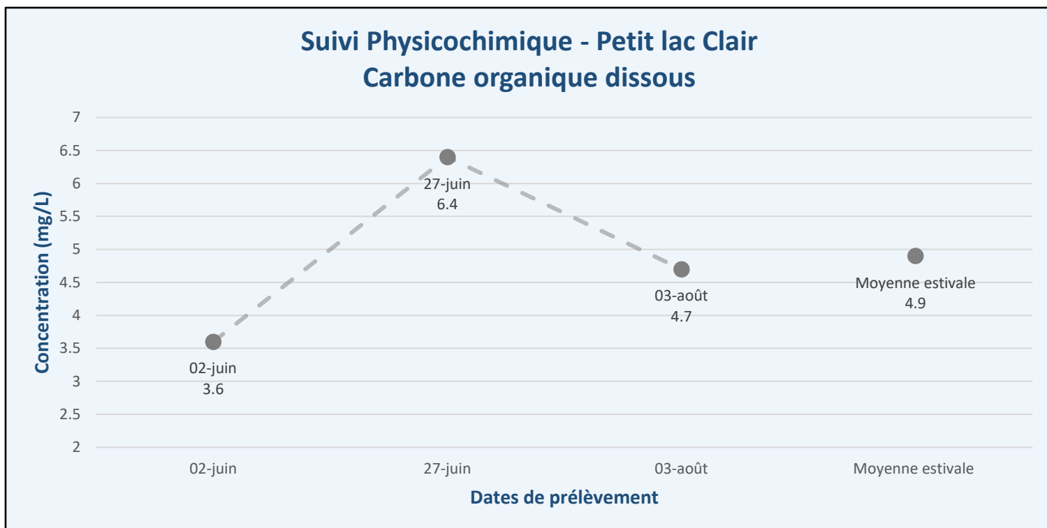
Figure 7 - Résultats – Suivi physicochimique 2021 (COD) – Petit lac Clair (PLC1)
