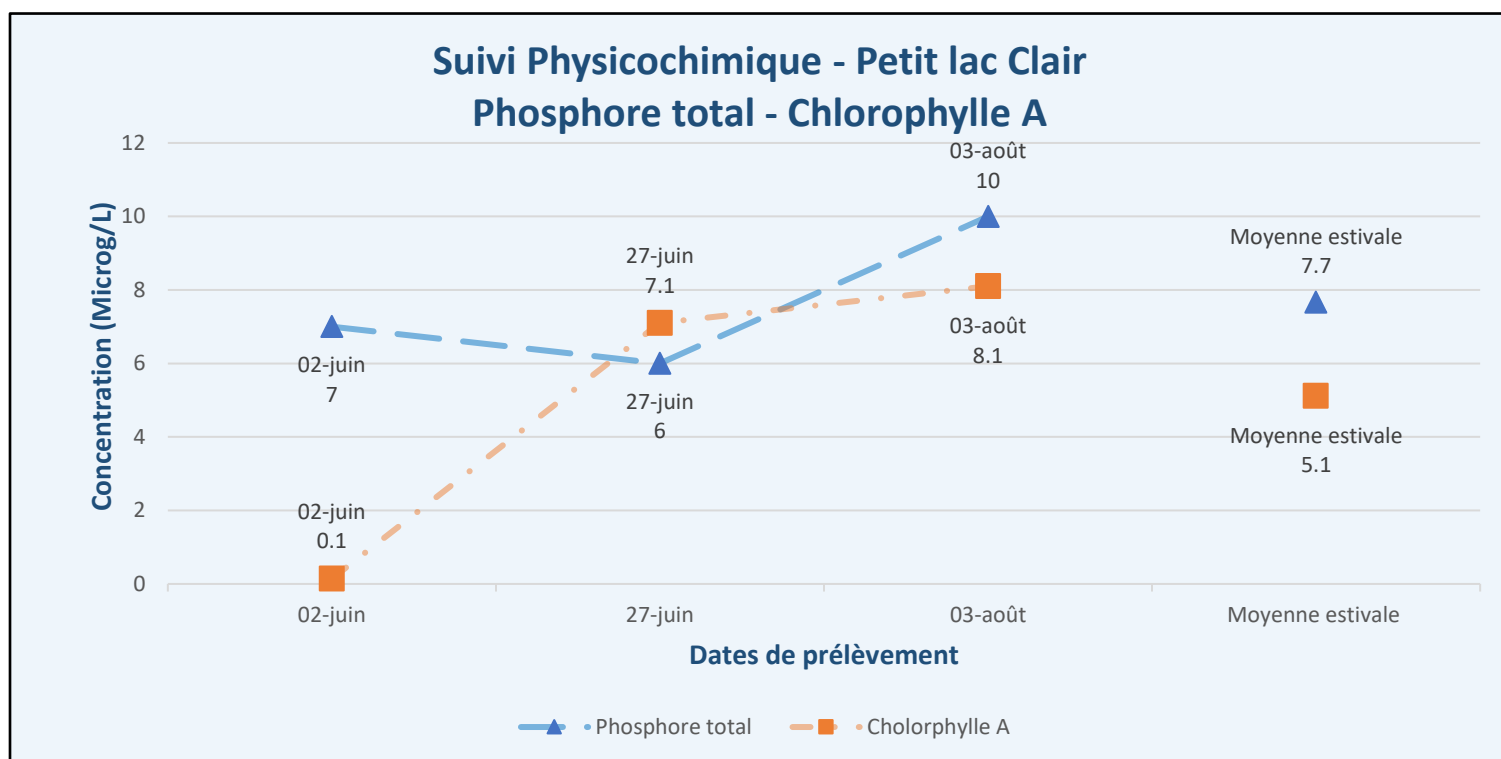
Figure 5 - Résultats – Suivi physicochimique 2021 (PT, Chla) – Petit lac Clair (PLC1)
