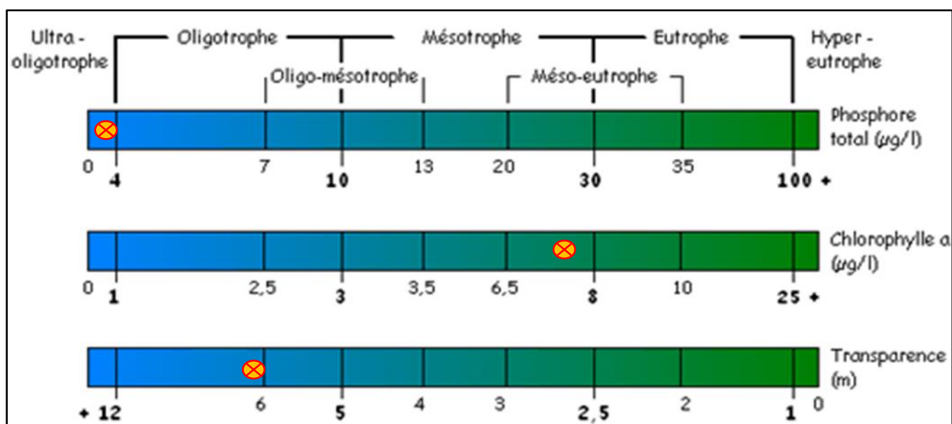
Figure 9 - État trophique 2021 - Lac des Épinettes (EP1)
