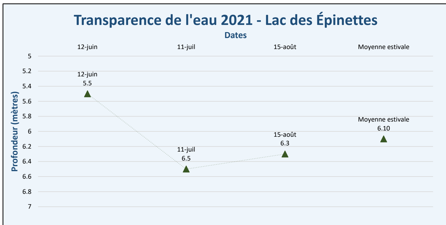
Figure 5 – Résultats transparence de l'eau 2021 - Lac des Épinettes
