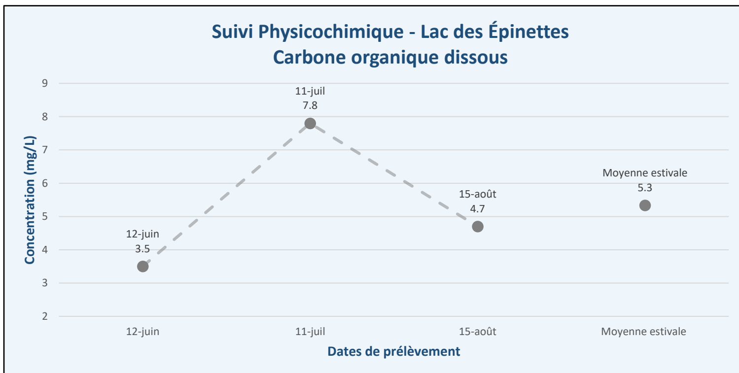
Figure 7 - Résultats – Suivi physicochimique 2021 (COD) - Lac des Épinettes (EP1)
