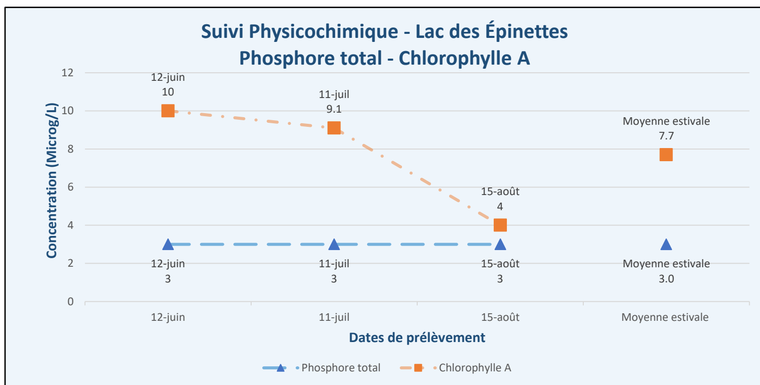
Figure 6 - Résultats – Suivi physicochimique 2021 (PT, Chla) – Lac des Épinettes (EP1)
