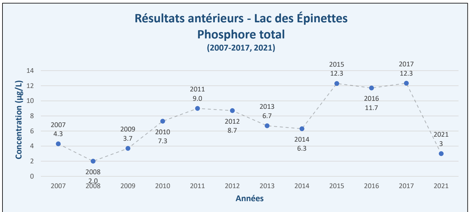
Figure 8 – Résultats antérieurs – Phosphore total - Lac des Épinettes
