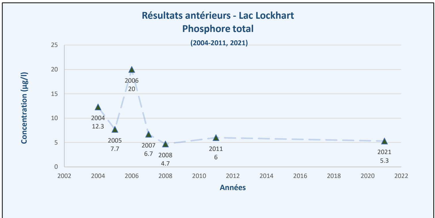
Figure 8 – Résultats antérieurs – Phosphore total – Chlorophylle A – Lac Lockhart (LK1)
