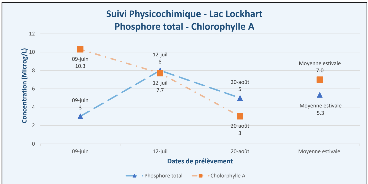
Figure 6 – Résultats – Suivi physicochimique 2021 (PT, Chla) – Lac Lockhart (LK1)
