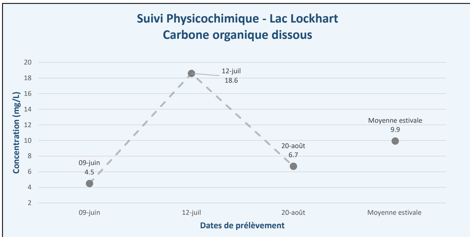
Figure 7 – Résultats – Suivi physicochimique 2021 (COD) – Lac Lockhart (LK1)
