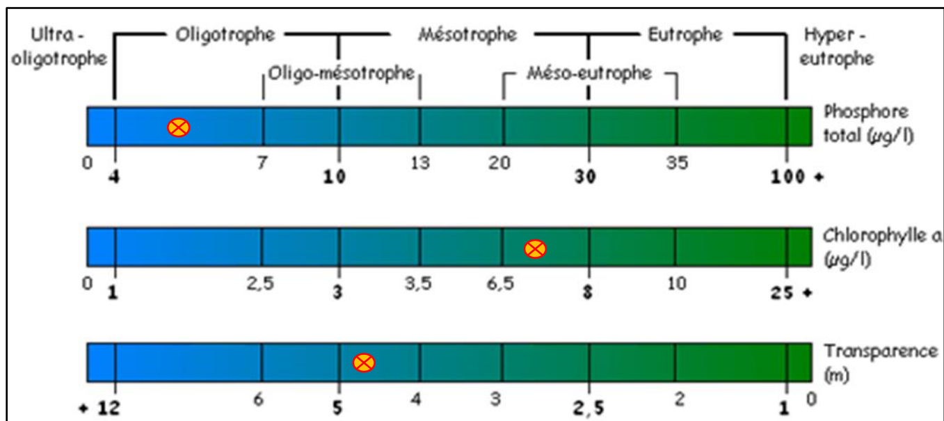
Figure 9 - État trophique 2021 - Lac Lockhart (LK1)
