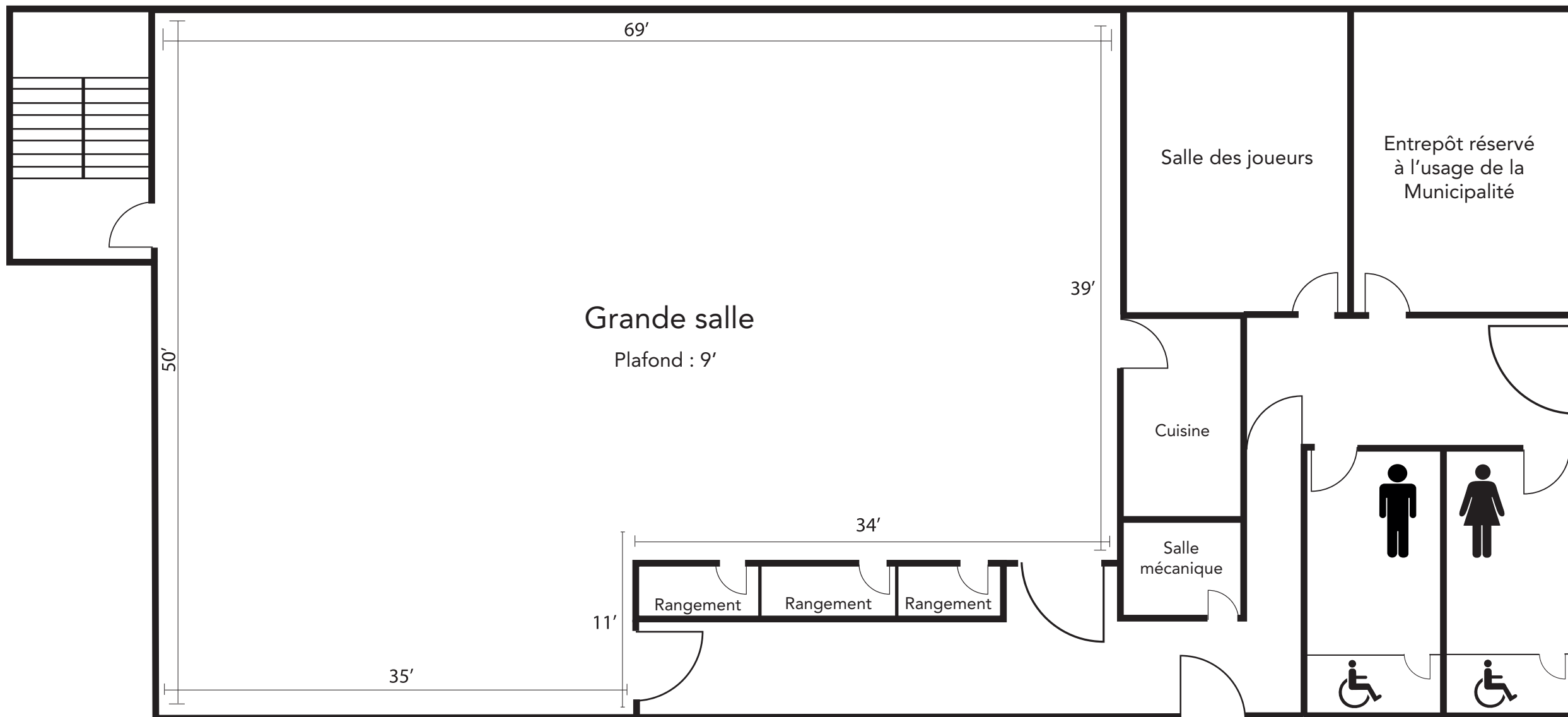
Plan du rez-de-chaussée
