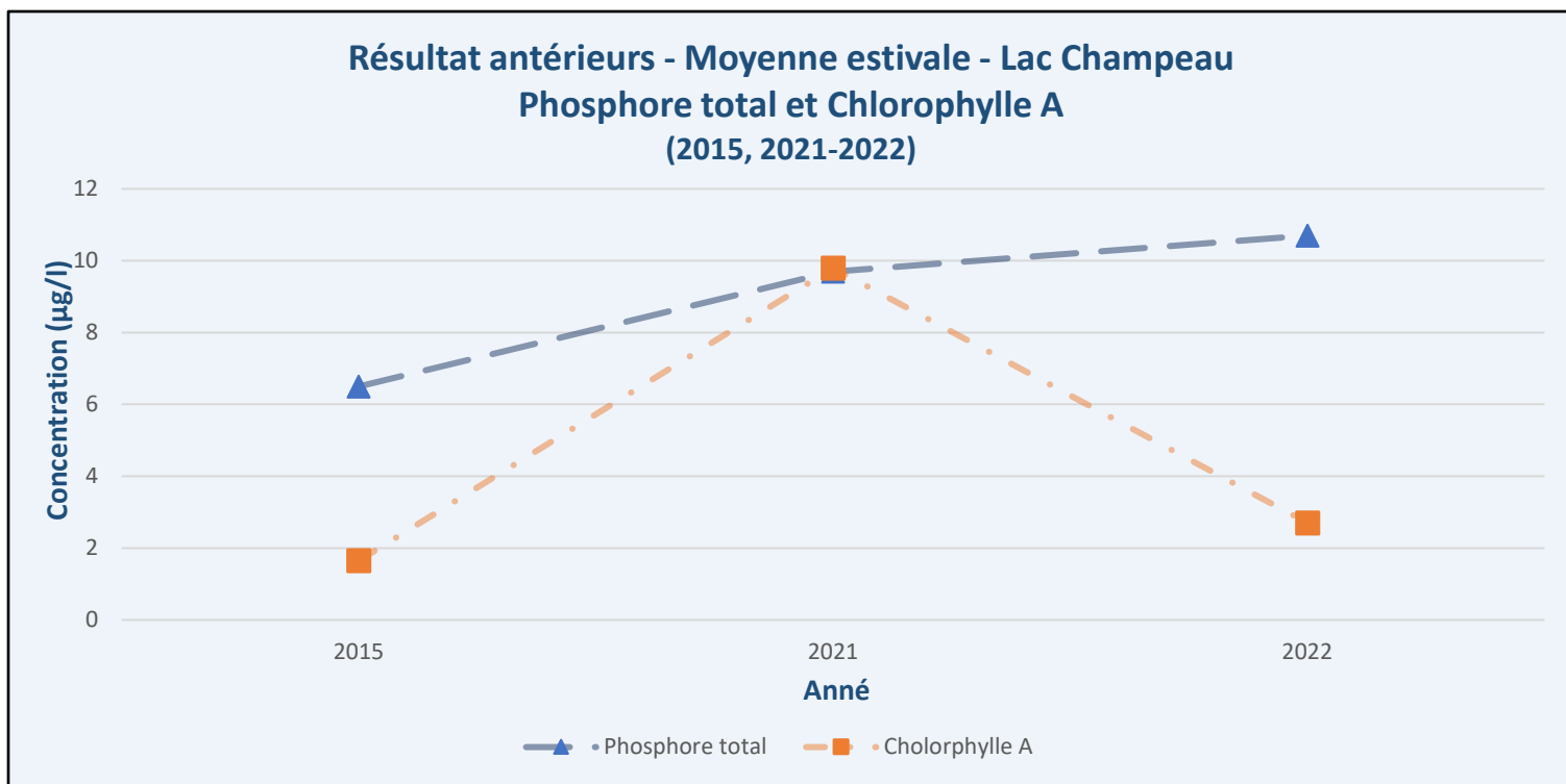
Figure 9 – Résultats antérieurs – Suivi physicochimique (PT, Chla) – Lac Champeau
