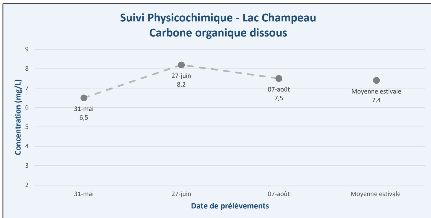
Figure 7 – Résultats – Suivi physicochimique 2022 (COD) – Lac Champeau (CP1)
