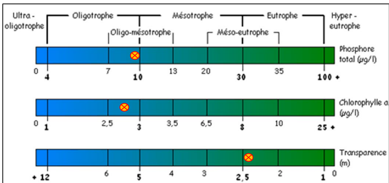
Figure 10 – État trophique 2022 – Station 1 – Lac Champeau (CP1)
