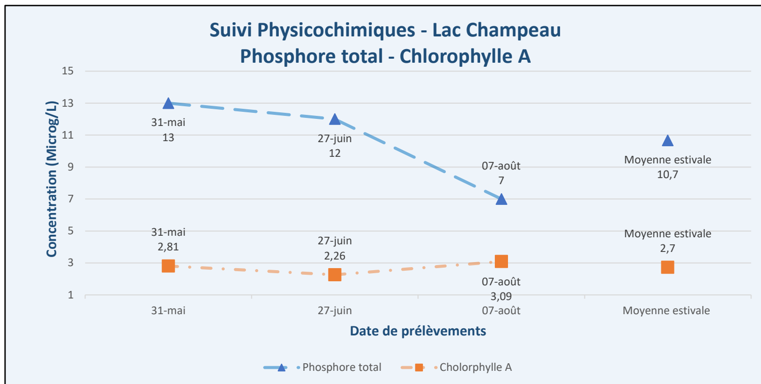
Figure 6 – Résultats – Suivi physicochimique 2022 (PT, Chla) – Lac Champeau (CP1)
