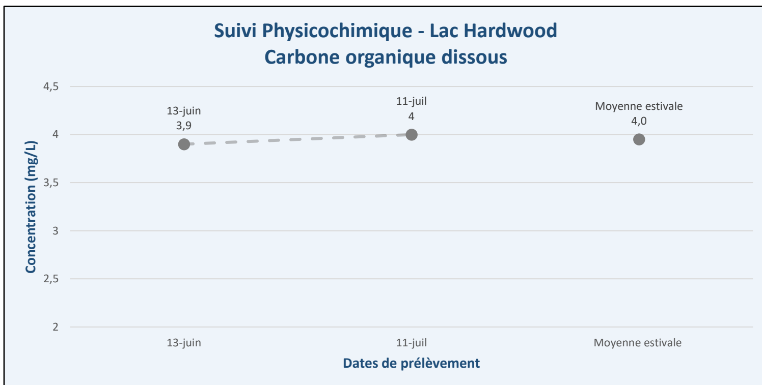
Figure 6 - Résultats – Suivi physicochimique 2022 (COD) - Lac Hardwood (HW1)
