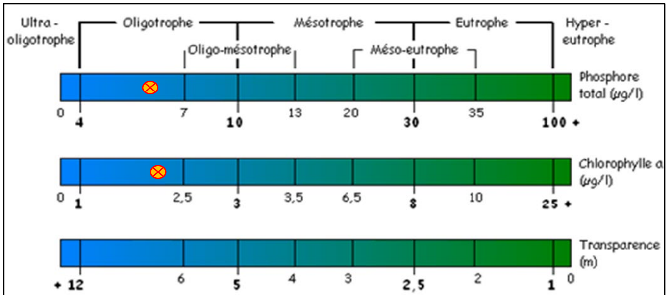
Figure 8 - État trophique 2022 - Lac Hardwood (HW1)
