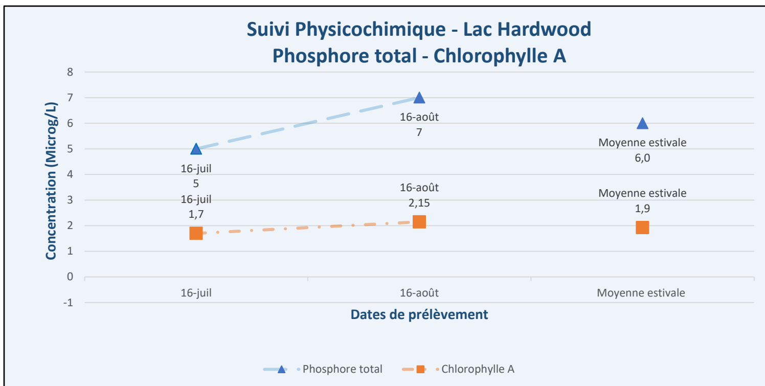
Figure 5 - Résultats – Suivi physicochimique 2022 (PT,Chla) – Lac Hardwood (HW1)
