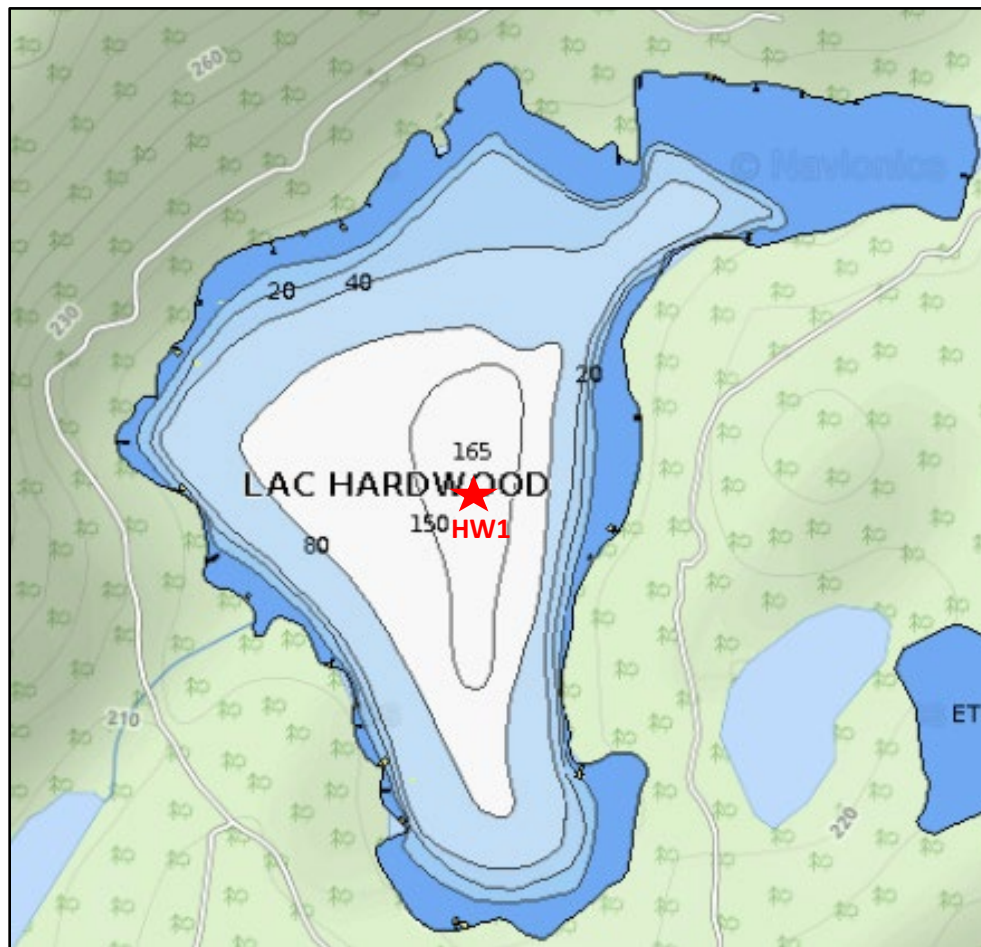
Figure 4 – Carte bathymétrique du lac Hardwood (Navionics, 2021)
