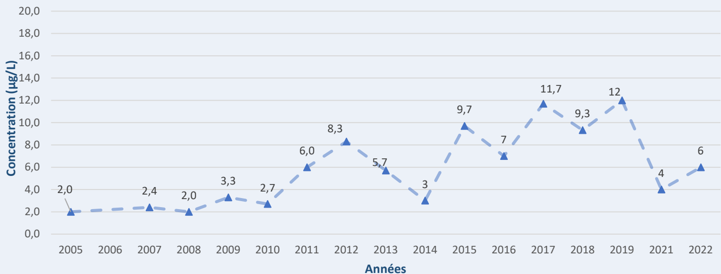
Figure 7 – Résultats antérieurs – Lac Hardwood (HW1)
