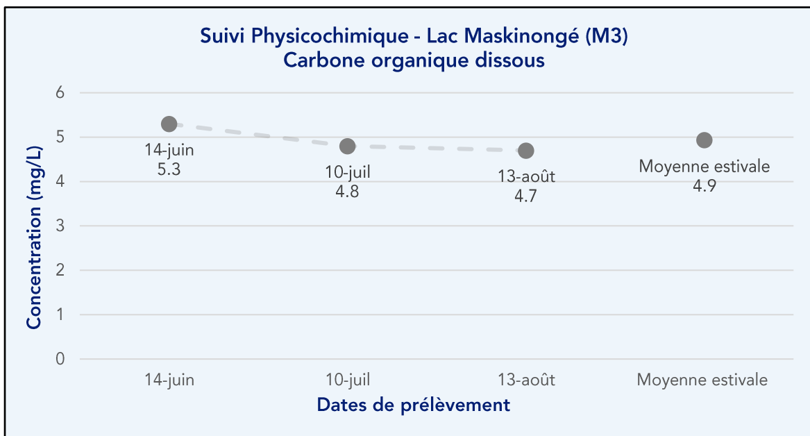
Figure 11 - Résultats – Suivi physicochimique 2024 (PT, COD) – Lac Maskinongé (M3)
