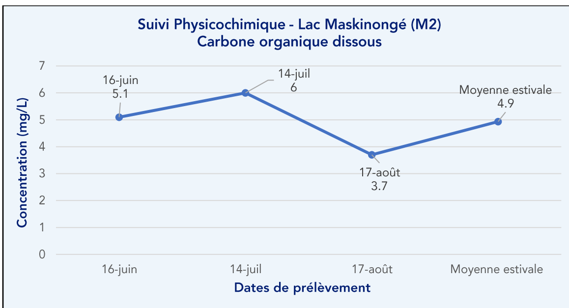
Figure 9 - Résultats – Suivi physicochimique 2024 (PT, COD) – Lac Maskinongé (M2)
