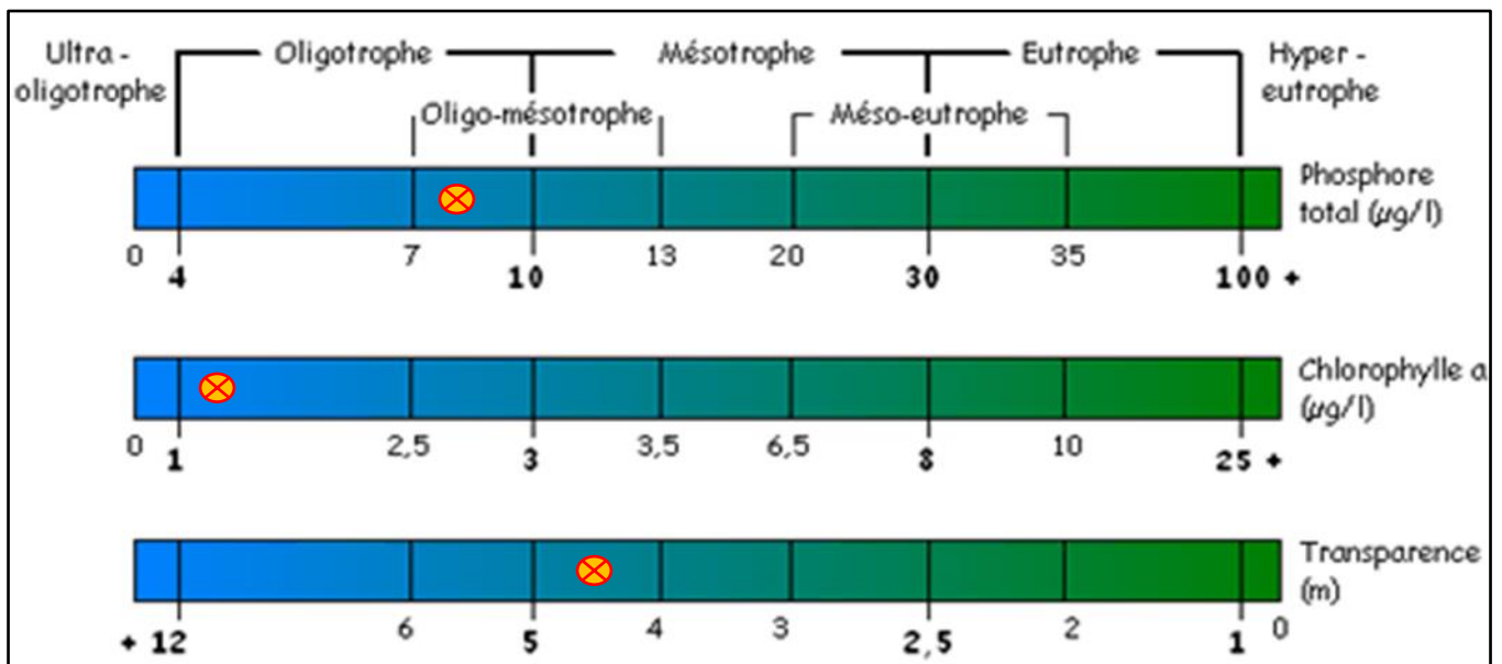
Figure 16 - État trophique 2024 - Station 3 – Lac Maskinongé (M3)
