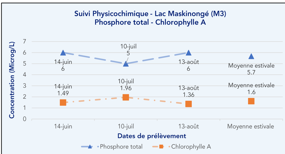
Figure 10 - Résultats – Suivi physicochimique 2024 (PT, Chla) – Lac Maskinongé (M3)
