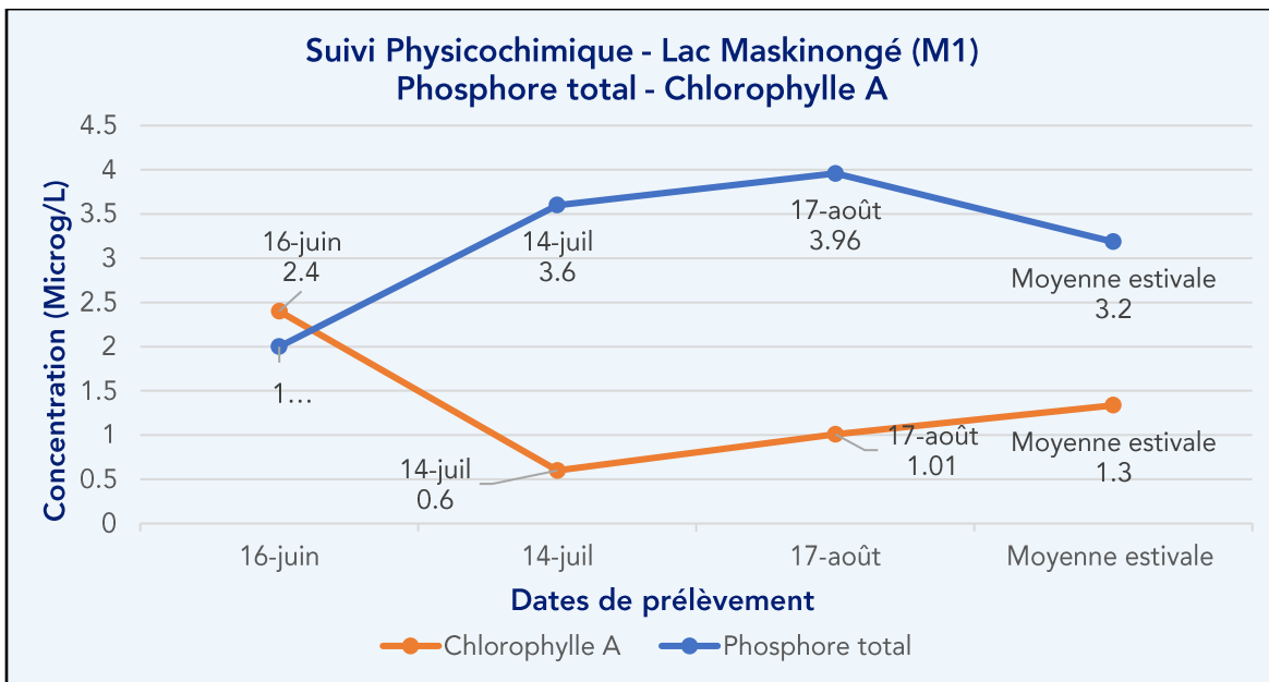
Figure 6 - Résultats – Suivi physicochimique 2024 (PT, Chla) – Lac Maskinongé (M1)
