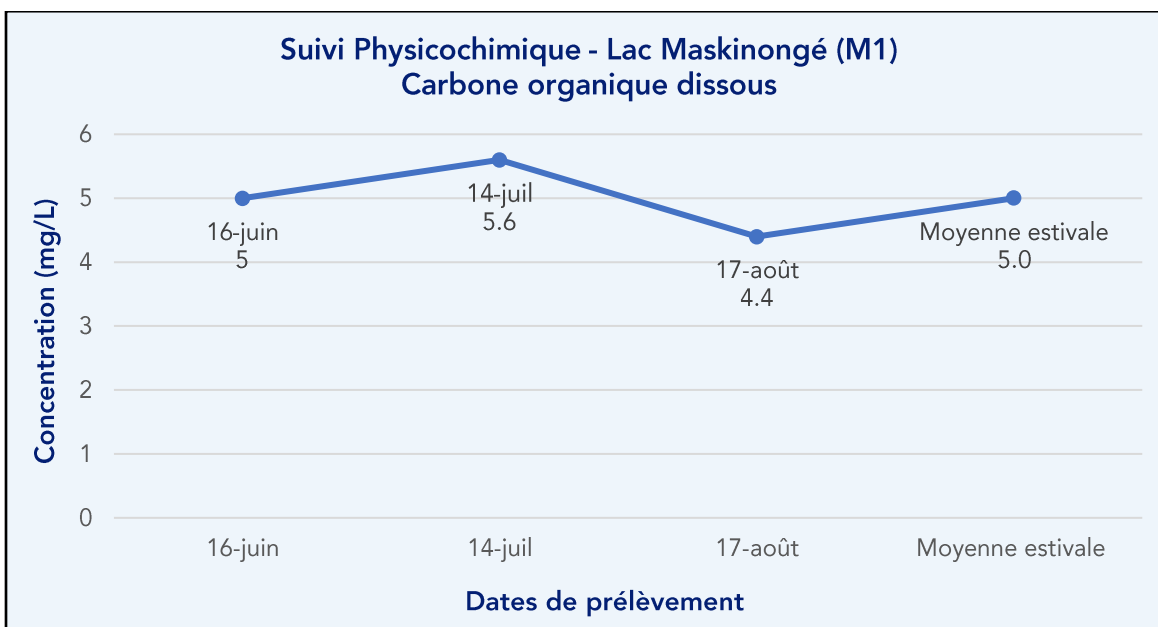
Figure 7 - Résultats – Suivi physicochimique 2024 (COD) - Lac Maskinongé (M1)
