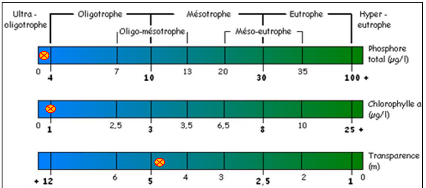
Figure 15 - État trophique 2024 - Station 2 – Lac Maskinongé (M2)
