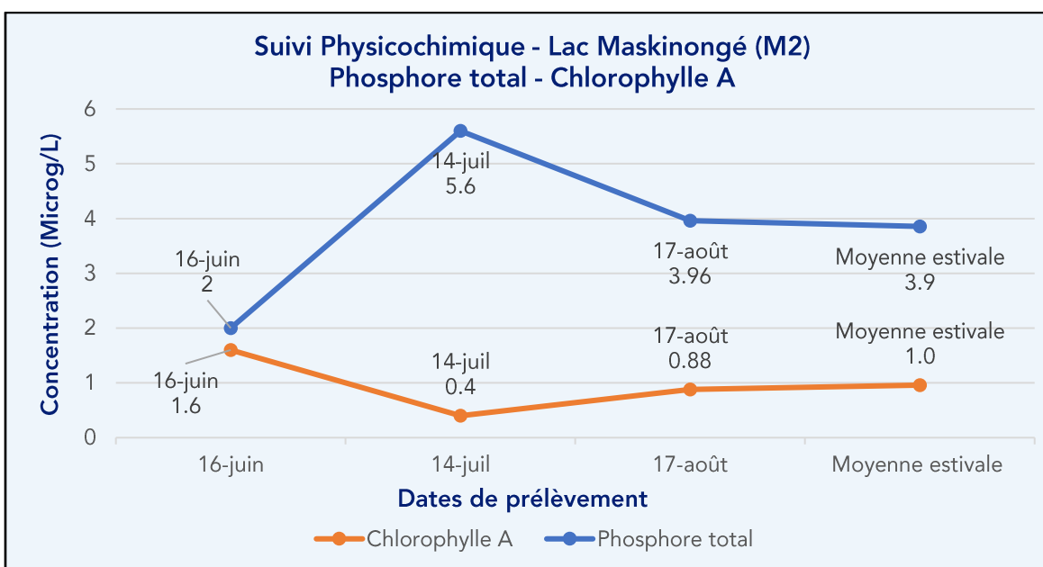
Figure 8 - Résultats – Suivi physicochimique 2024 (PT, Chla) – Lac Maskinongé (M2)
