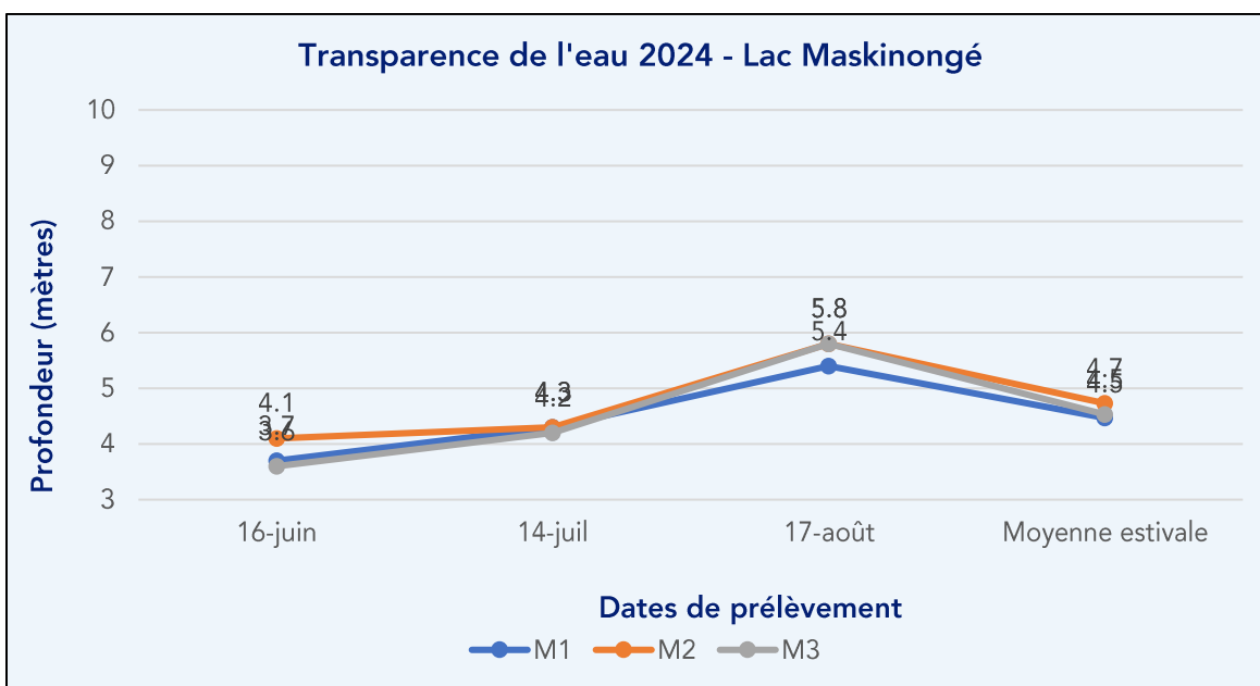
Figure 5 – Résultats transparence de l'eau 2024 – Lac Maskinongé
