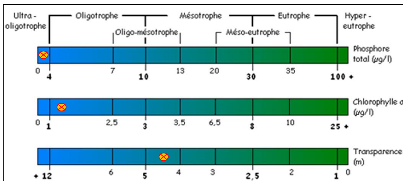
Figure 14 - État trophique 2024 - Station 1 – Lac Maskinongé (M1)
