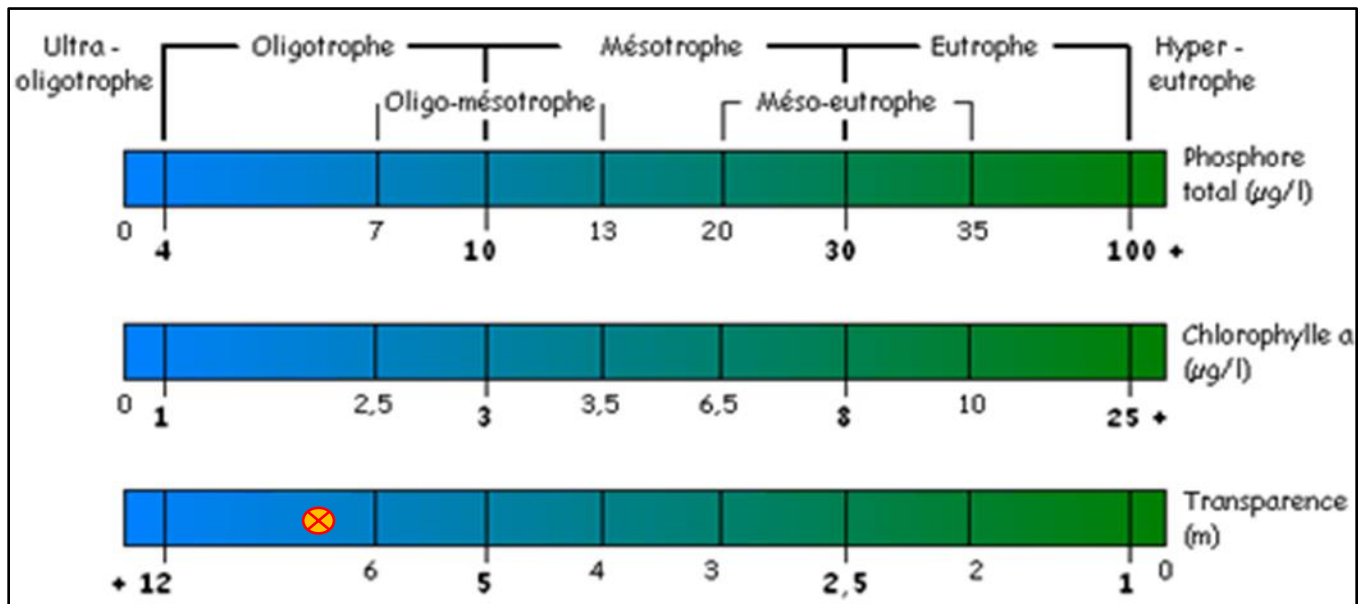
Figure 19 —État trophique 2024 —Station 4 —Lac Rhéaume (R4)
