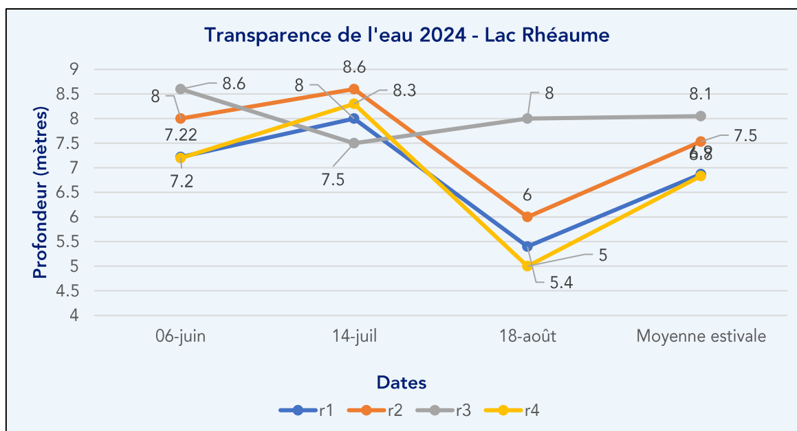
Figure 6 — Résultats transparence de l'eau 2024 — Lac Rhéaume
