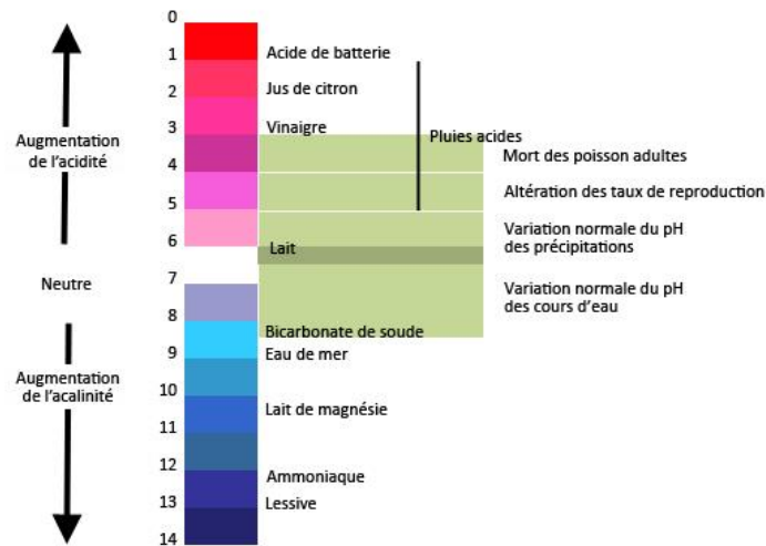
Figure 4 — Échelle du pH
