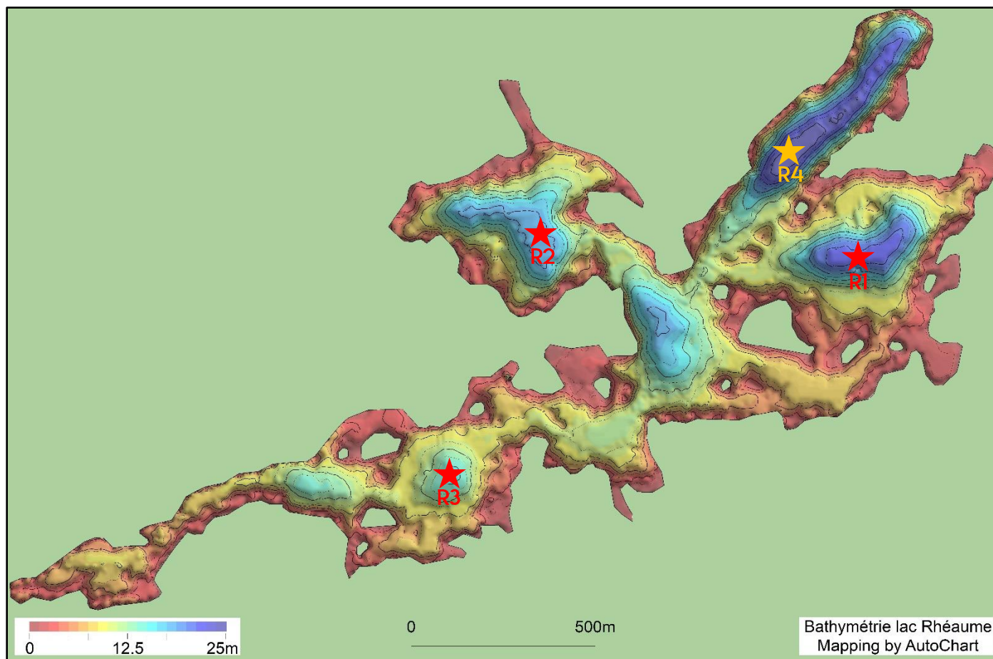
Figure 5 — Carte bathymétrique du lac Rhéaume (Fédération des lacs de Val-des-Monts, 2020)
