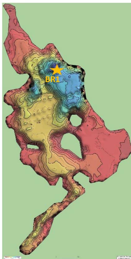
Figure 4 – Carte bathymétrique du lac Brassard, FDLVDM, 2018
