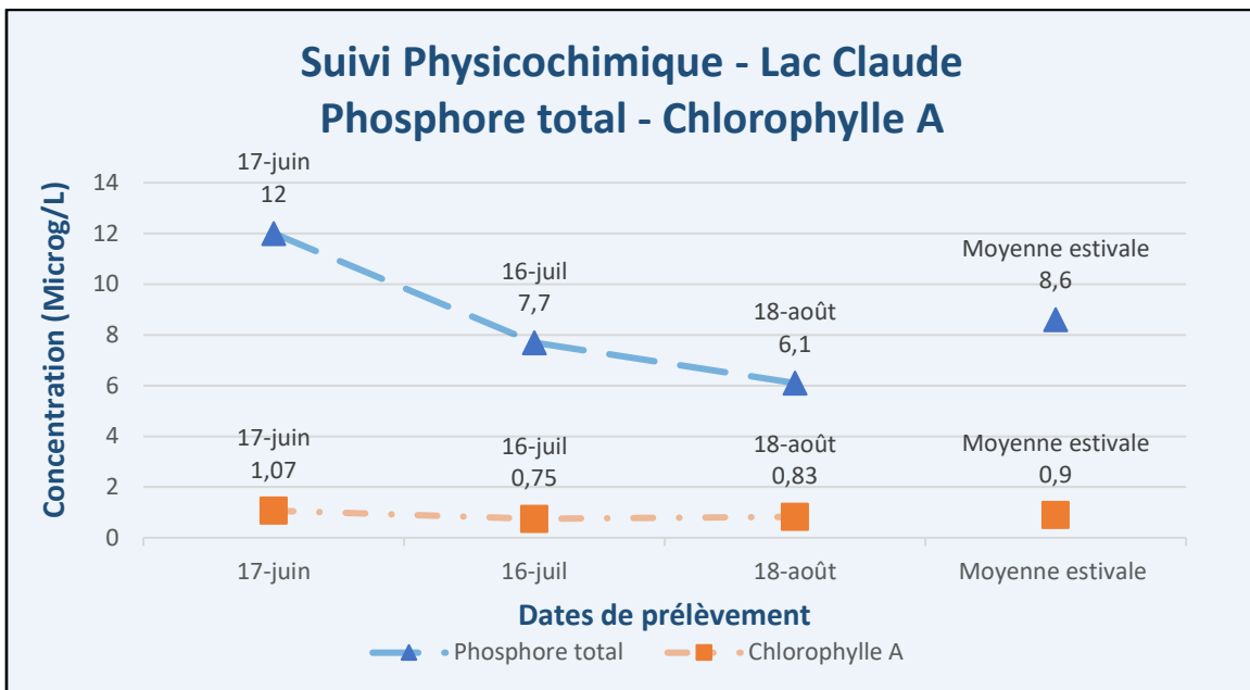
Figure 7 – Résultats – Suivi physicochimique 2025 (PT, Chla) – Lac Claude (CL1)
