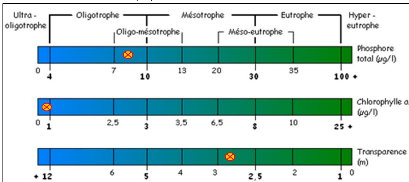
Figure 10 – État trophique 2025 – Lac Claude (CL1)
