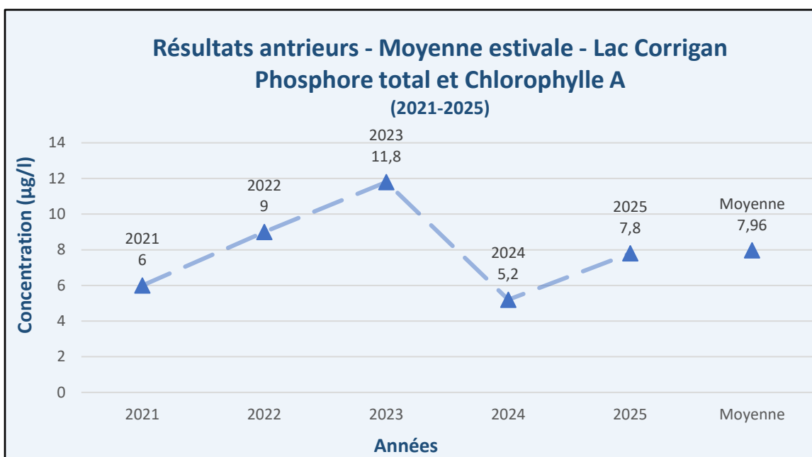
Figure 7 – Résultats antérieurs – Phosphore total – Lac Corrigan (C1)
