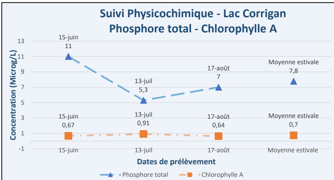
Figure 5 – Résultats – Suivi physicochimique 2025 (PT, Chla) – Lac Corrigan (C1)
