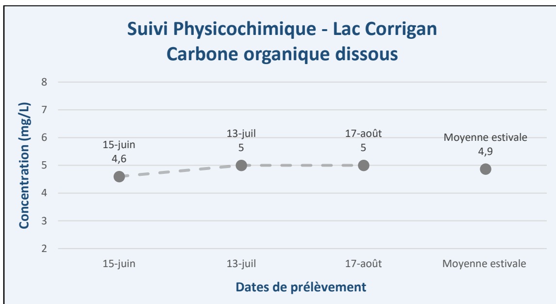
Figure 6 – Résultats – Suivi physicochimique 2025 (COD) – Lac Corrigan (C1)
