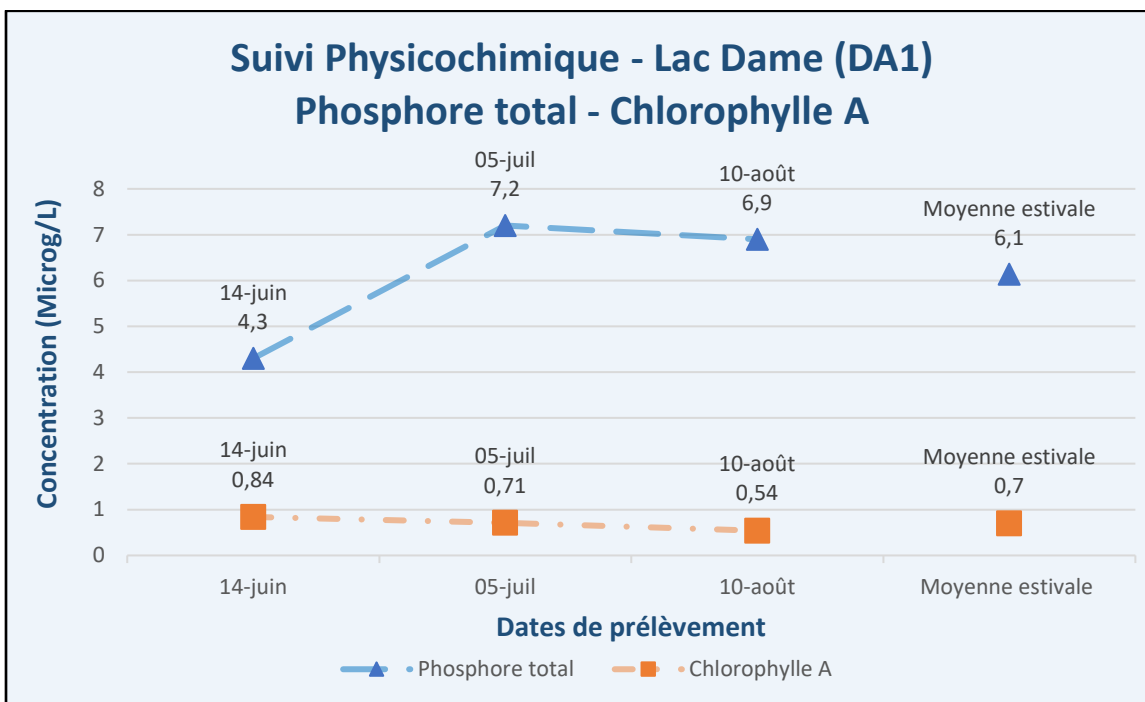
Figure 6 – Résultats – Suivi physicochimique 2025 (PT, Chla) – Lac Dame (DA1)
