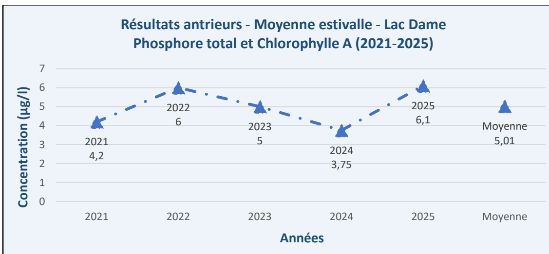
Figure 12 – Résultats antérieurs – Phosphore total et Chlorophylle A – Lac Dame
