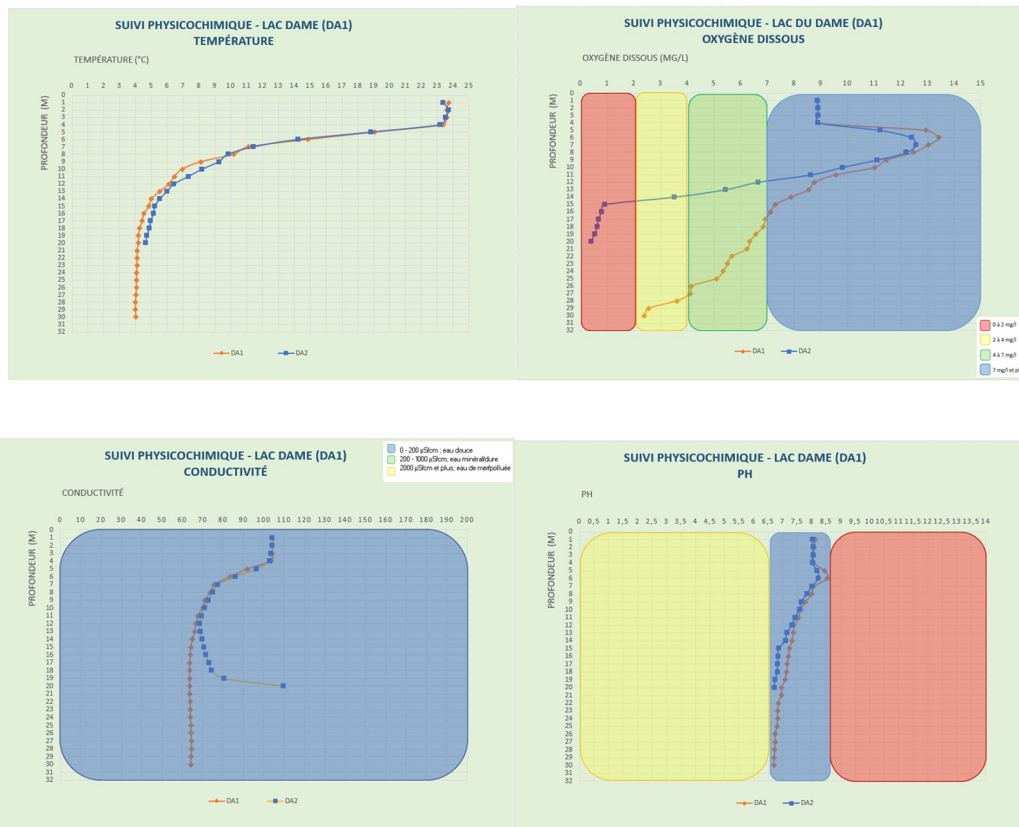
Figure 10 – Résultats – Profils physicochimiques 2024 – Lac Dame (DA1)
