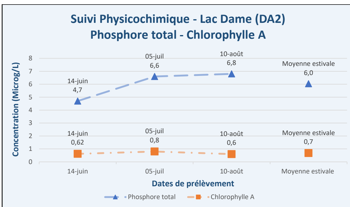
Figure 8 – Résultats – Suivi physicochimique 2025 (PT, Chla) – Lac Dame (DA2)
