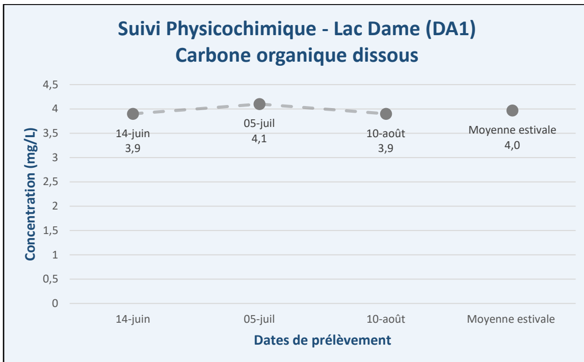
Figure 7 – Résultats – Suivi physicochimique 2025 (COD) - Lac Dame (DA1)
