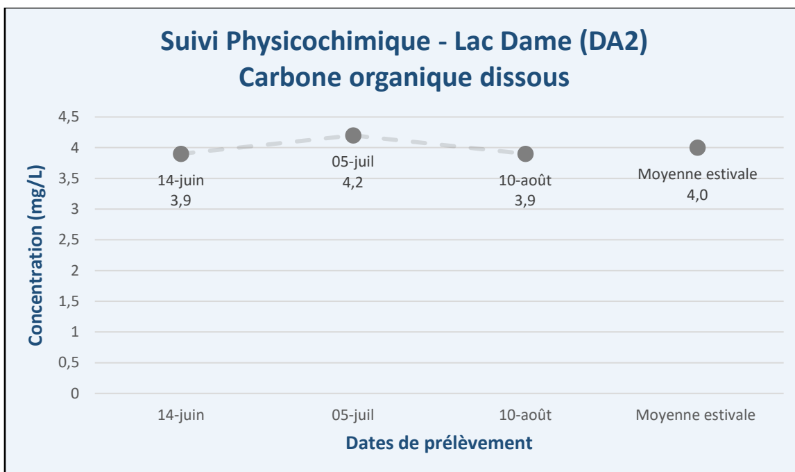
Figure 9 – Résultats – Suivi physicochimique 2025 (COD) – Lac Dame (DA2)
