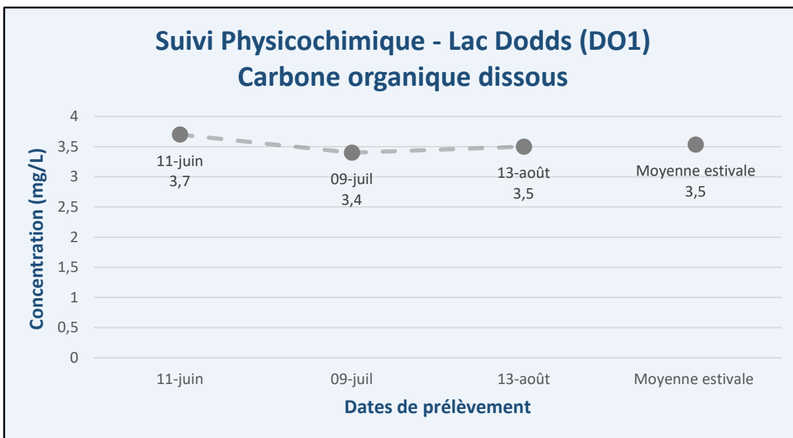
Figure 8 – Résultats – Suivi physicochimique 2025 (COD) – Lac Dodds (DO1)
