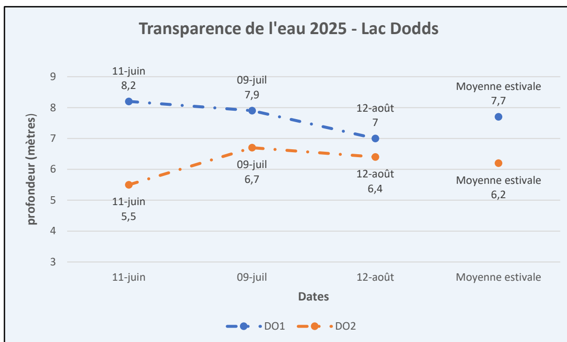
Figure 6 – Résultats – Transparence de l'eau 2025 – Lac Dodds
