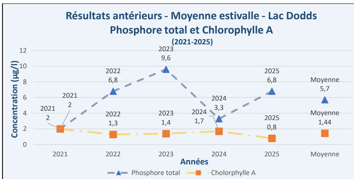
Figure 11 – Résultats antérieurs – Phosphore total – Chlorophylle A – Lac Dodds (DO1)
