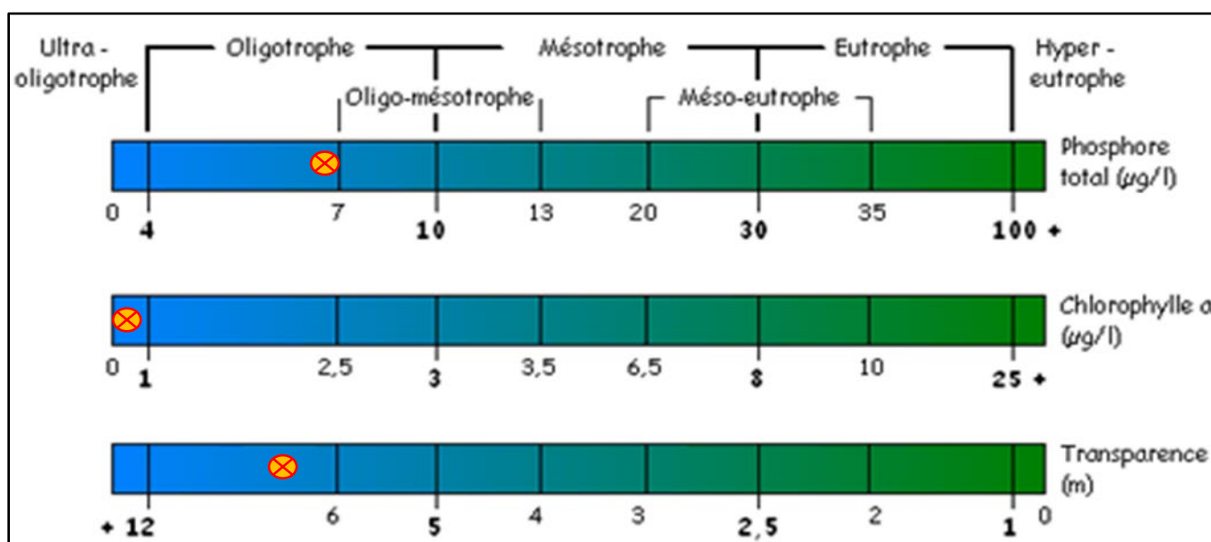
Figure 12 – État trophique 2025 – Station 1 – Lac Dodds (DOI)
