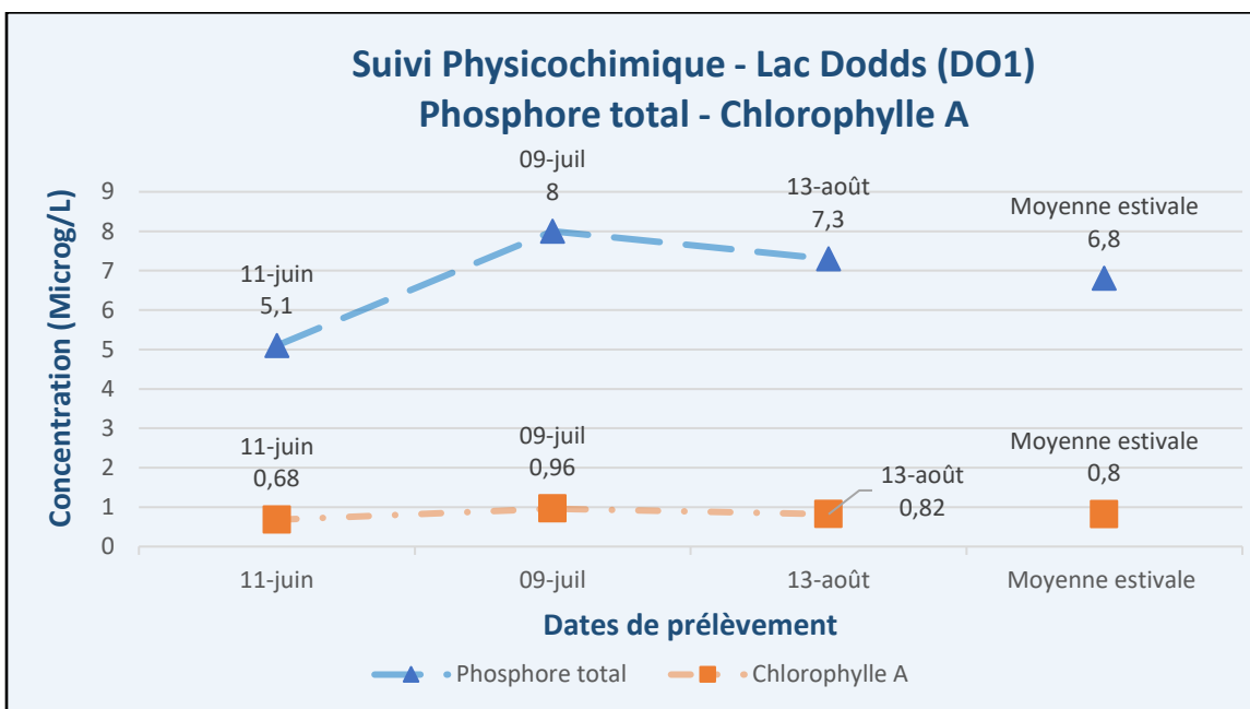
Figure 7 – Résultats – Suivi physicochimique 2025 (PT, Chla) – Lac Dodds (DO1)
