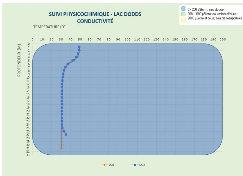
Figure 9 – Résultats – Profils physicochimiques 2024 – Lac Dodds (DO1)
