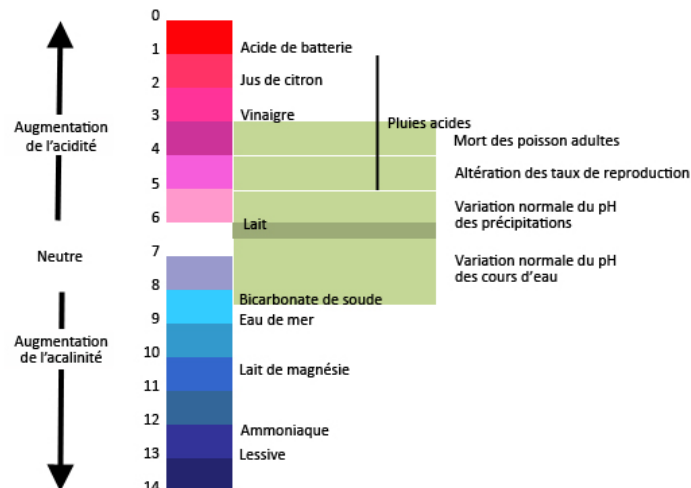
Figure 4 – Échelle du pH
