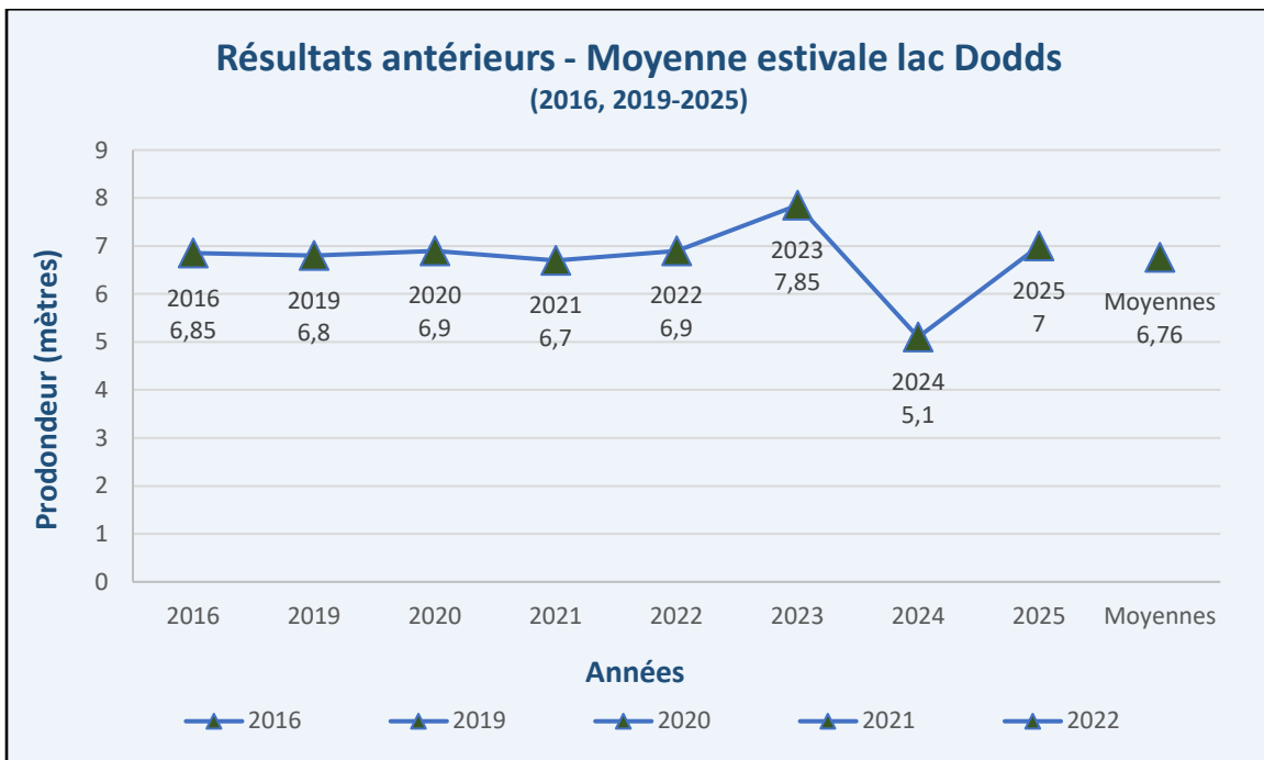
Figure 10 – Résultats antérieurs – Transparence de l'eau – Lac Dodds
