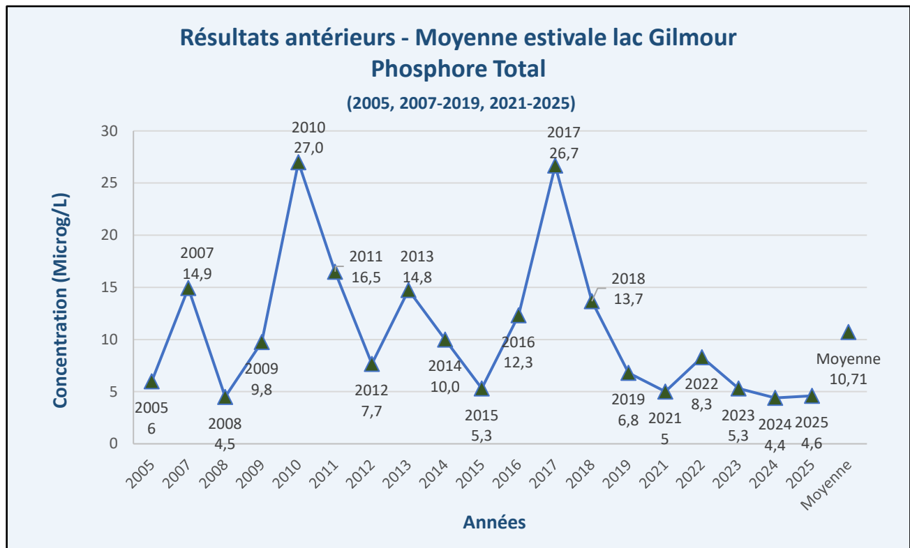
Figure 9 – Résultats antérieurs – Phosphore total – Lac Gilmour (GM1)
