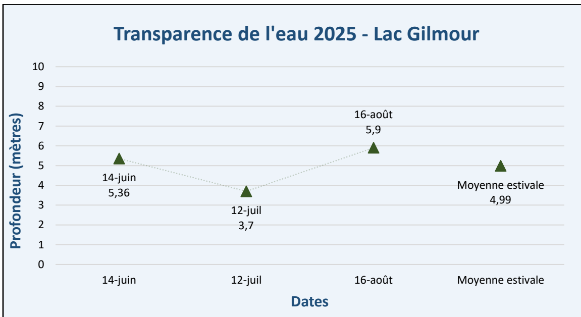
Figure 5 – Résultats – Transparence de l'eau 2025 – Lac Gilmour
