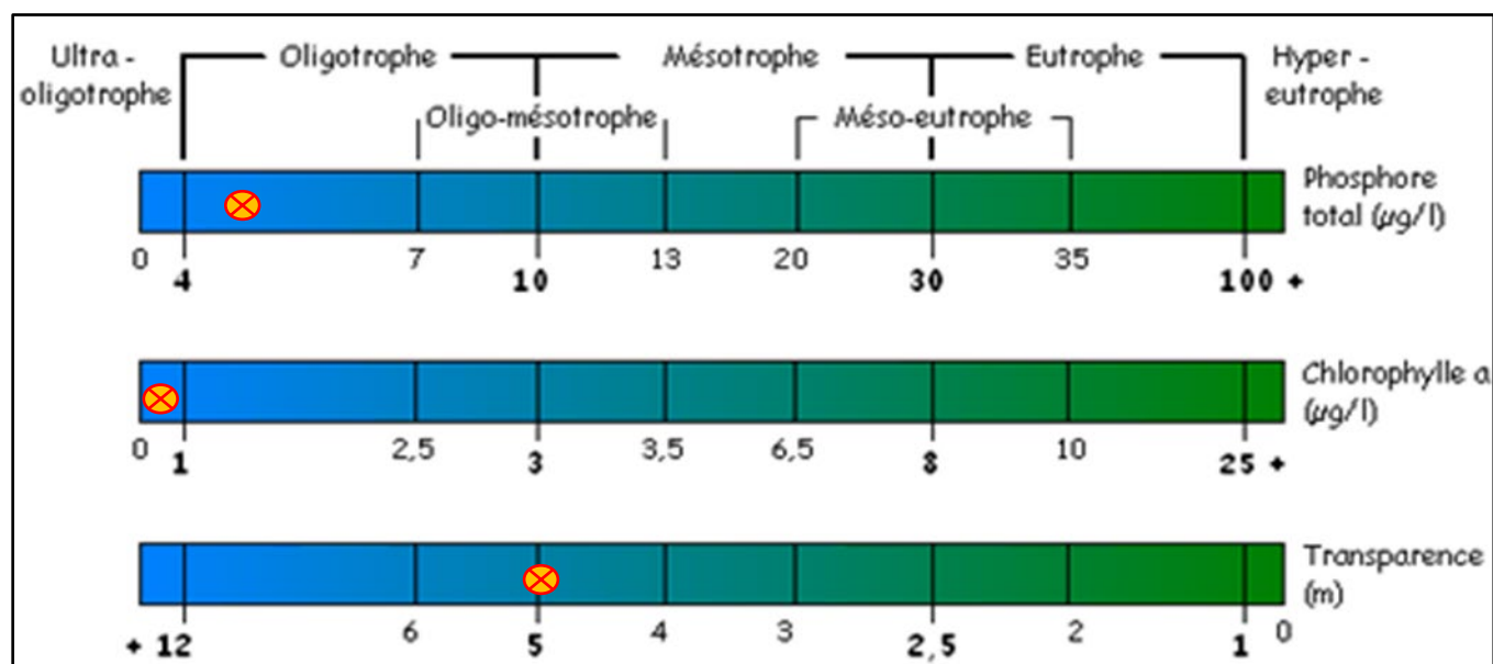
Figure 10 – État trophique 2025 – Lac Gilmour (GM1))
