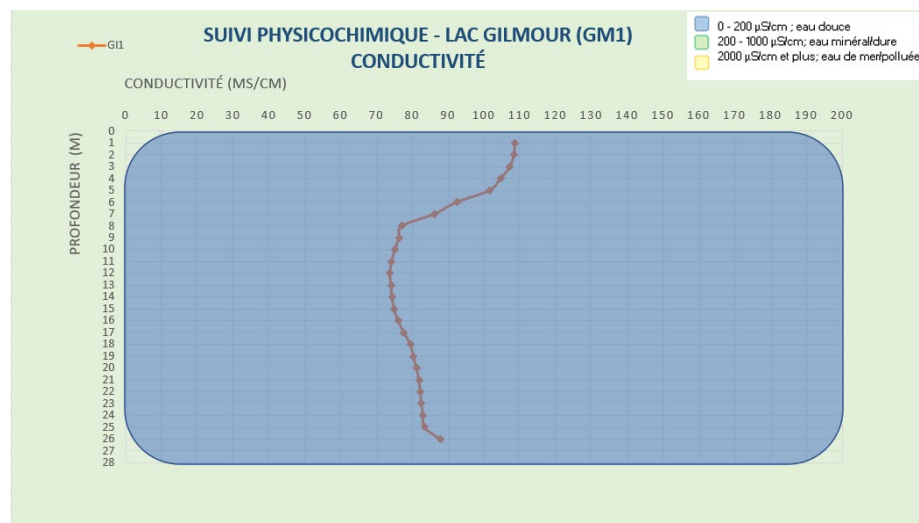
Figure 8 – Résultats – Profils physicochimiques 2024 – Lac Gilmour (GM1)
