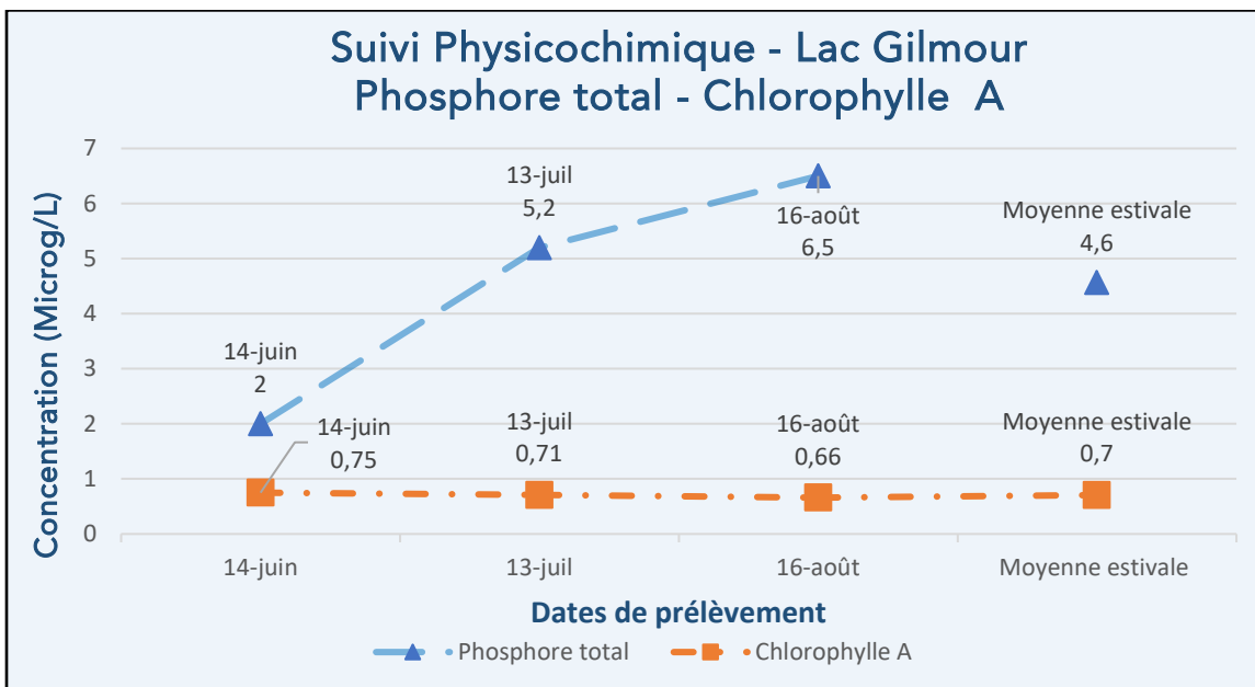
Figure 6 – Résultats – Suivi physicochimique 2025 (PT, Chla) – Lac Gilmour (GM1)
