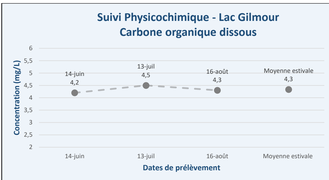
Figure 7 – Résultats – Suivi physicochimique 2025 (COD) – Lac Gilmour (GM1)
