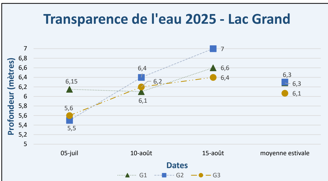
Figure 5 – Résultats – Suivi Transparence 2025 – Lac Grand (G1, G2, G3)
