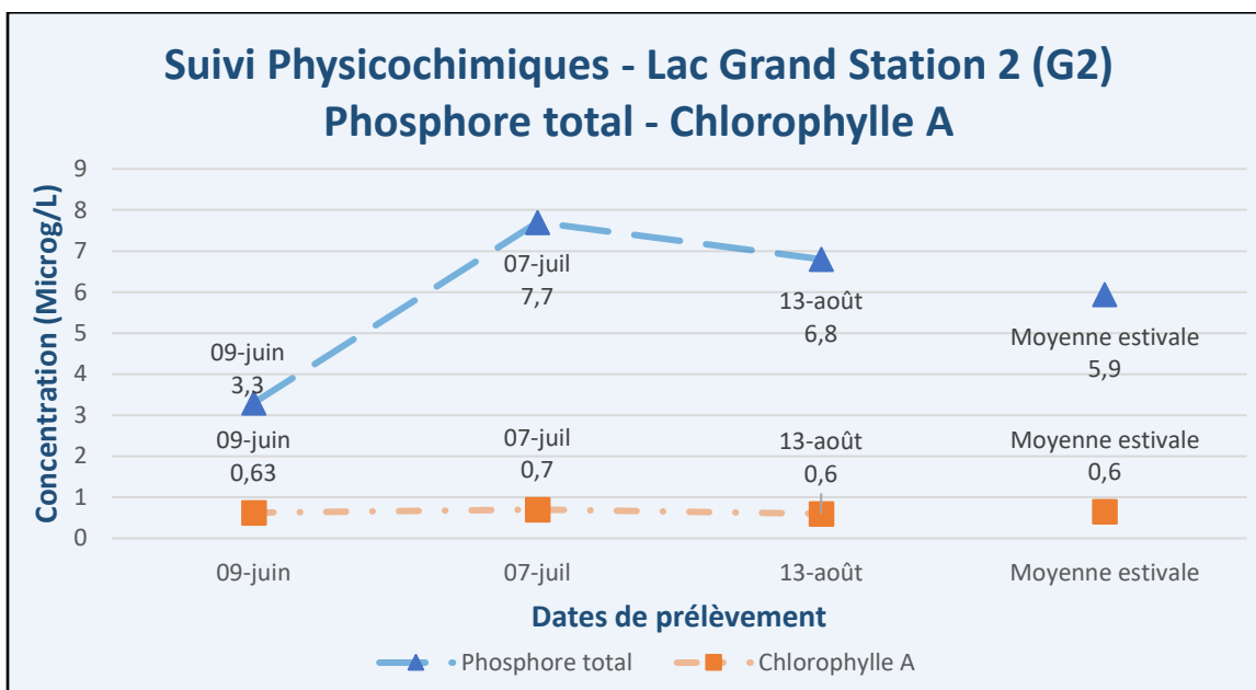
Figure 8 – Résultats – Suivi physicochimique 2025 (PT, Chla) – Lac Grand (G2)
