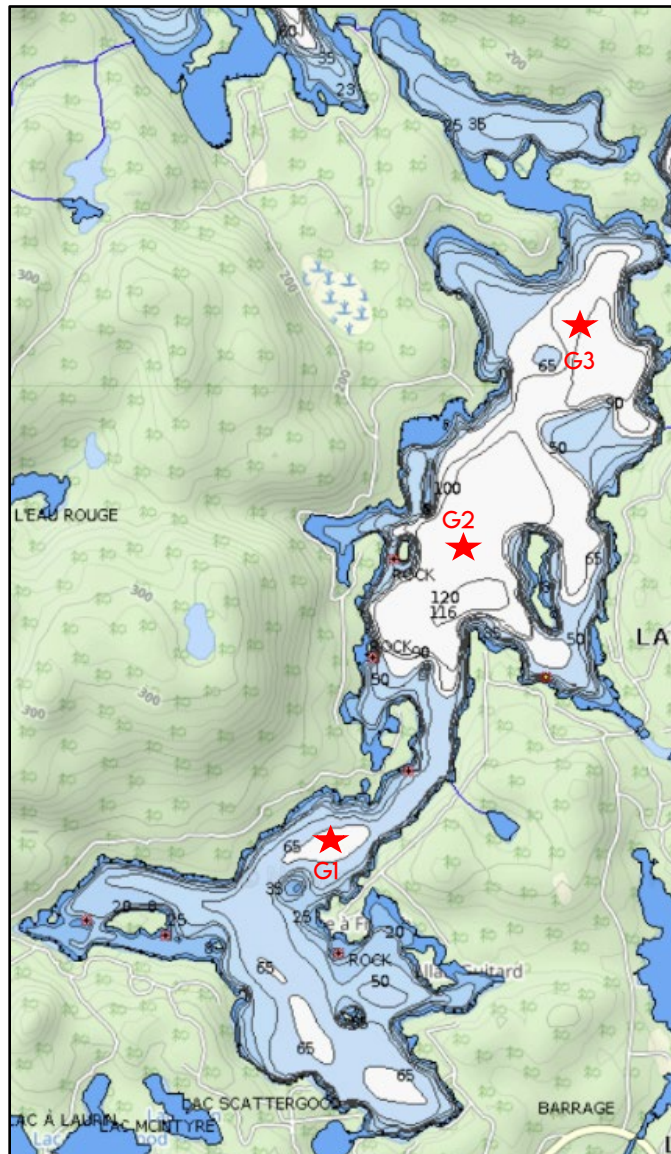
Figure 4 – Carte bathymétrique du lac Grand (Navionics, 2021)
