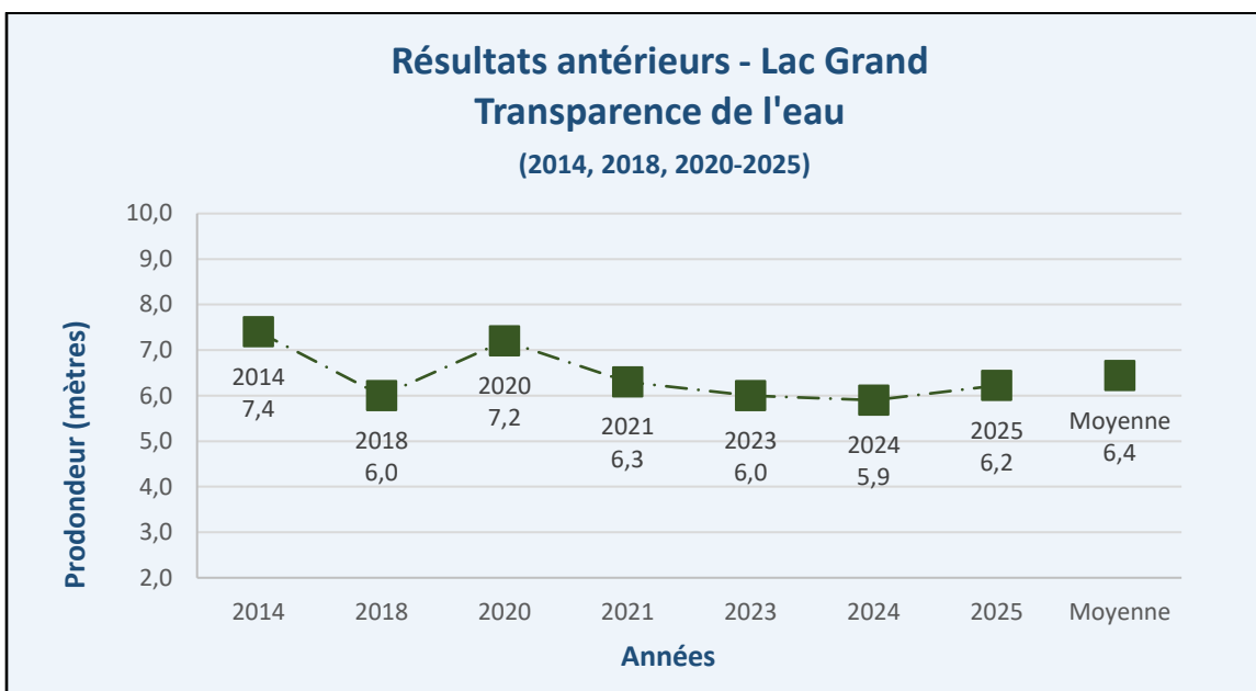
Figure 14 – Résultats antérieurs – Transparence de l'eau – Lac Grand
