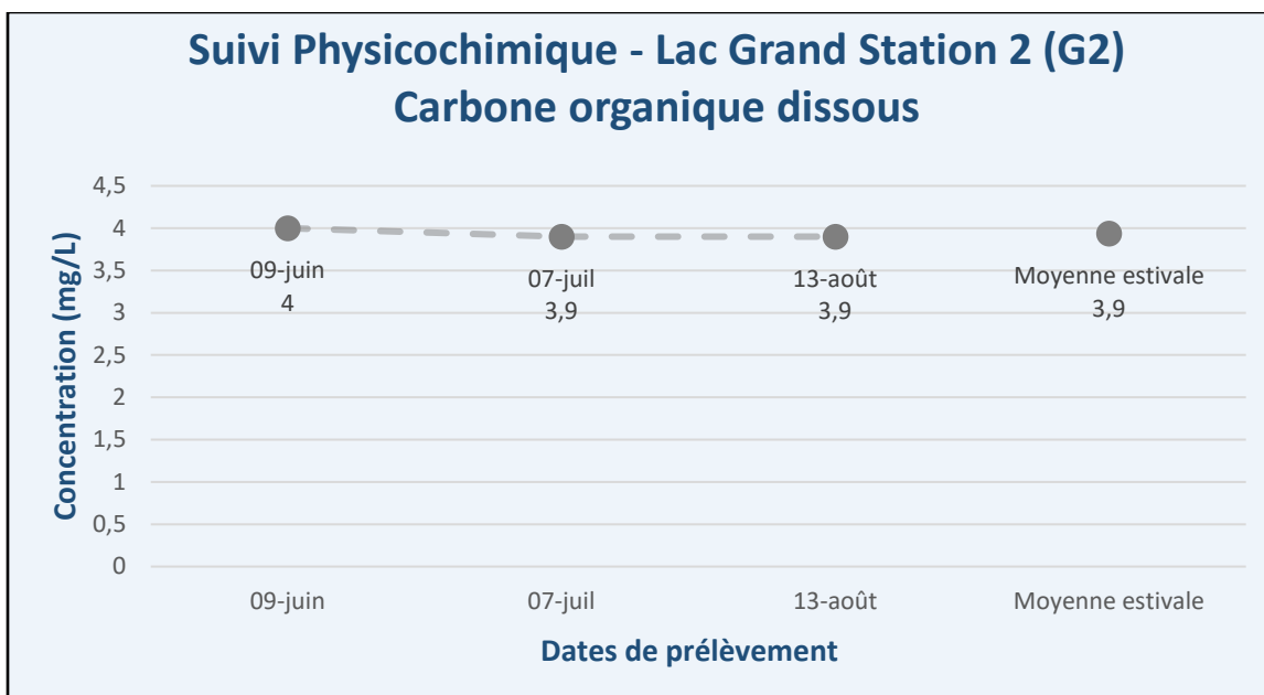
Figure 9 – Résultats – Suivi physicochimique 2025 (COD) – Lac Grand (G2)
