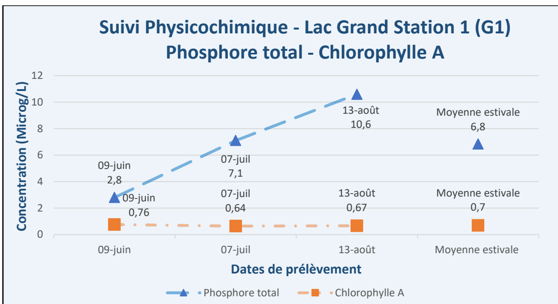
Figure 6 – Résultats – Suivi physicochimique 2025 (PT, Chla) – Lac Grand (G1)
