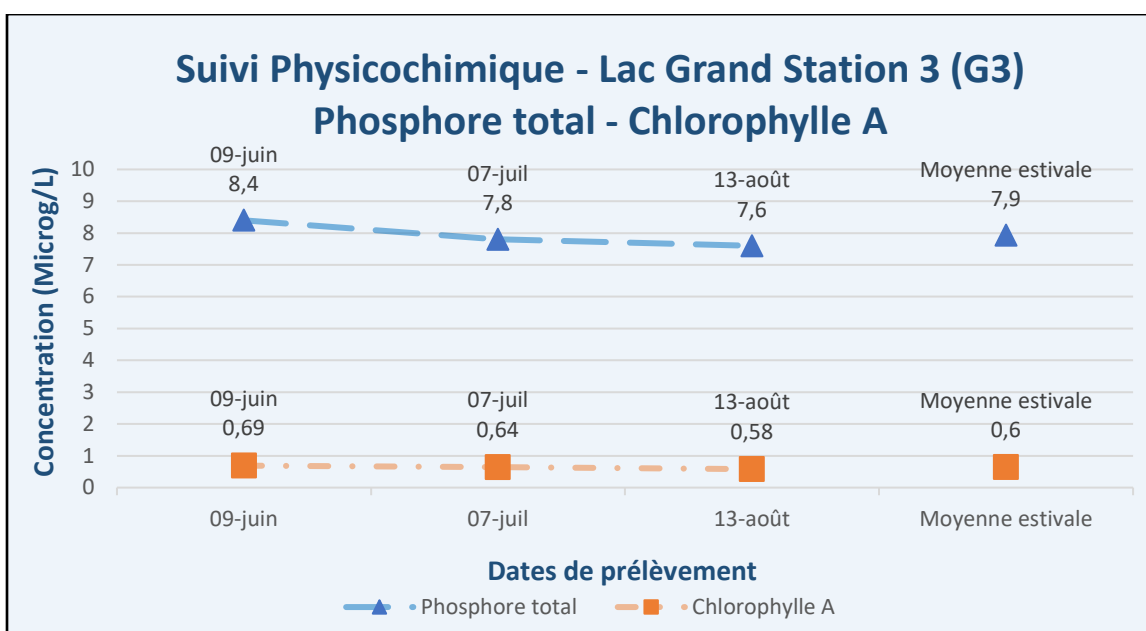
Figure 10 – Résultats – Suivi physicochimique 2025 (PT, Chla) – Lac Grand (G3)
