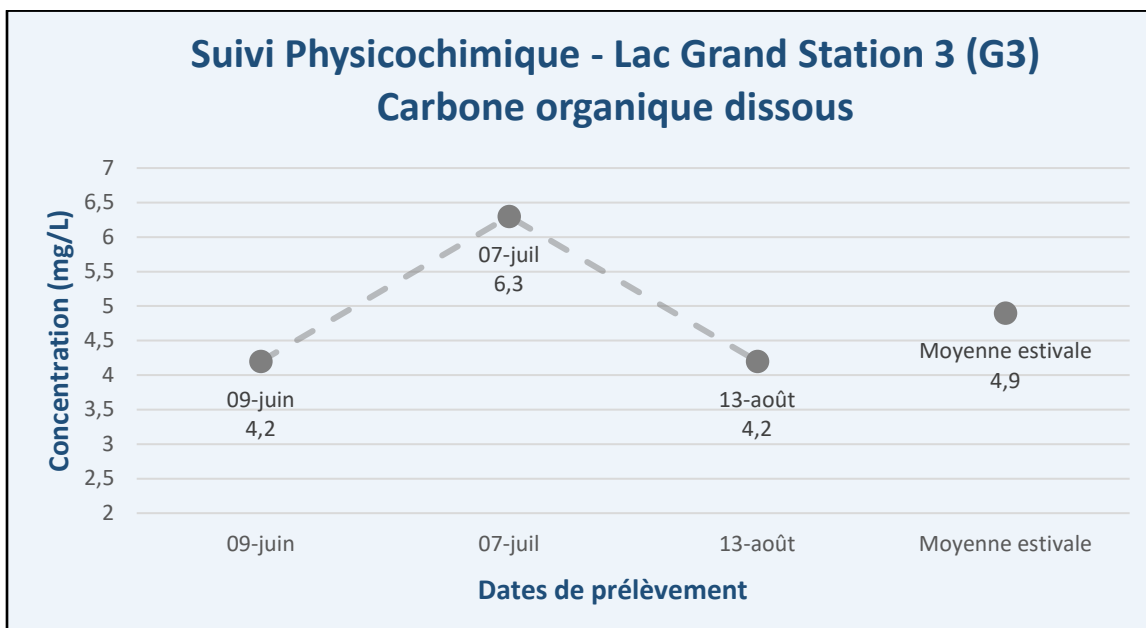
Figure 11 – Résultats – Suivi physicochimique 2025 (COD) – Lac Grand (G3)
