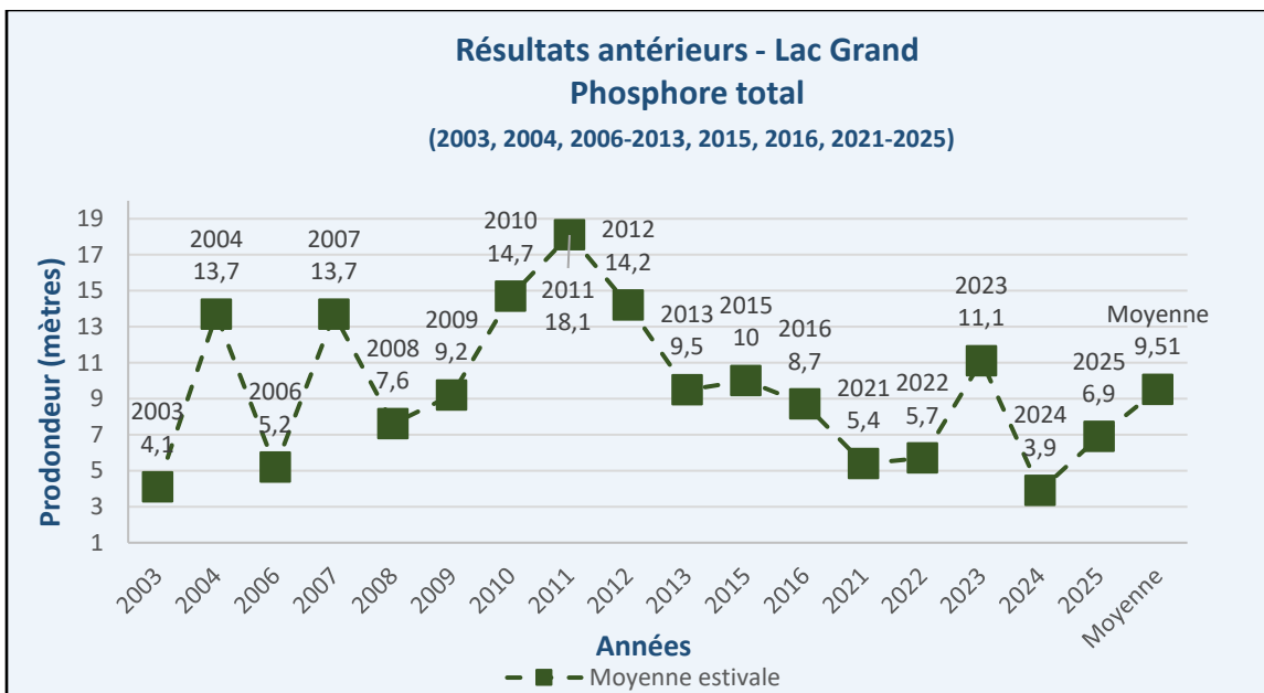
Figure 13 – Résultats antérieurs – Phosphore total – Lac Grand
