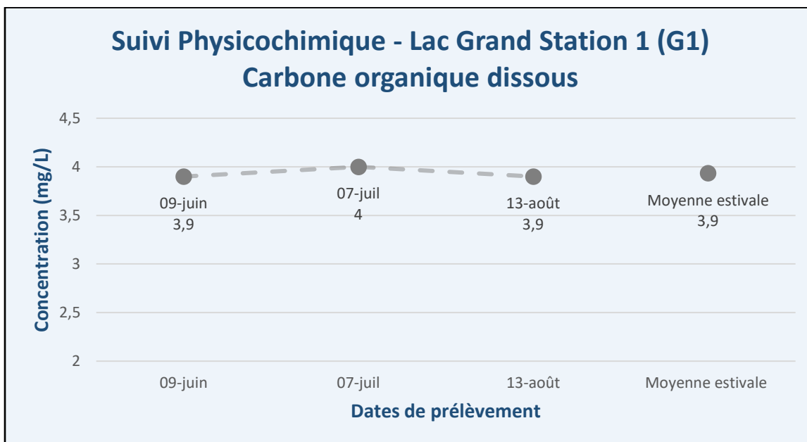
Figure 7 – Résultats – Suivi physicochimique 2025 (COD) – Lac Grand (G1)
