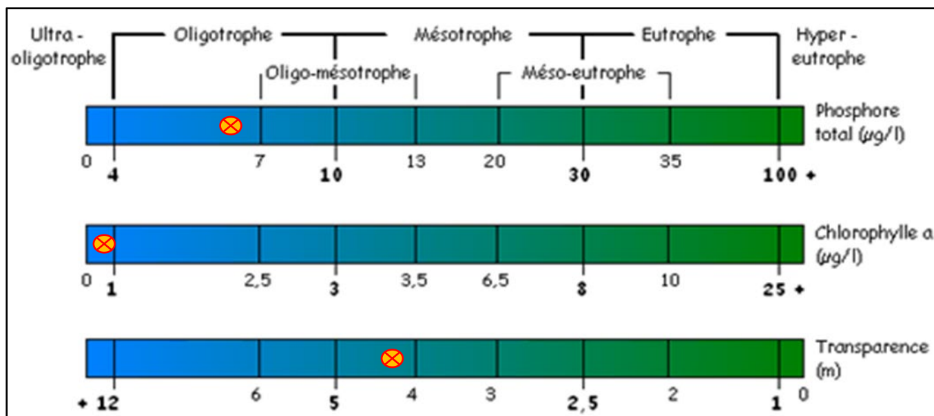
Figure 10 – État trophique 2025 – Lac Houston (Ho1)
