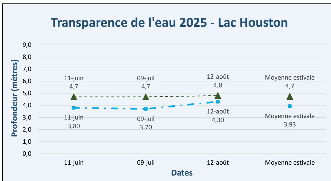
Figure 6 – Résultats – Transparence de l'eau 2025 – Lac Houston
