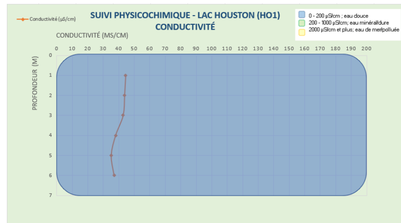
Figure 9 – Résultats – Profils physicochimiques 2025 – Lac Houston (Ho1)
