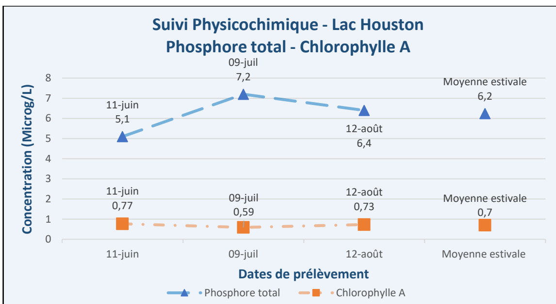
Figure 7 – Résultats – Suivi physicochimique 2025 (PT, Chla) – Lac Houston (Ho1)
