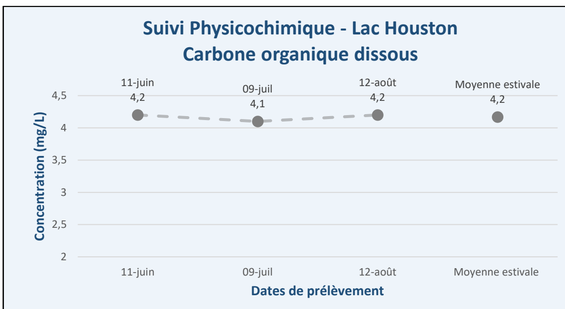
Figure 8 – Résultats – Suivi physicochimique 2025 (COD) – Lac Houston (Ho1)
