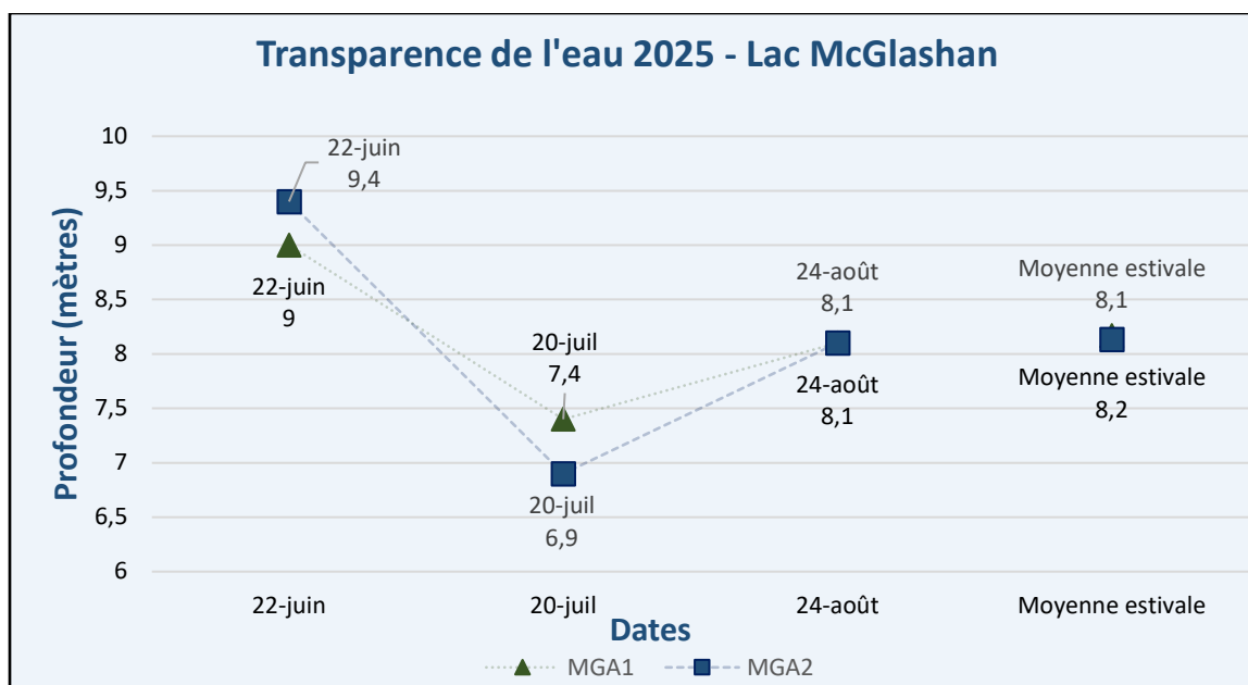
Figure 6 – Résultats – Transparence de l'eau 2025 – Lac McGlashan
