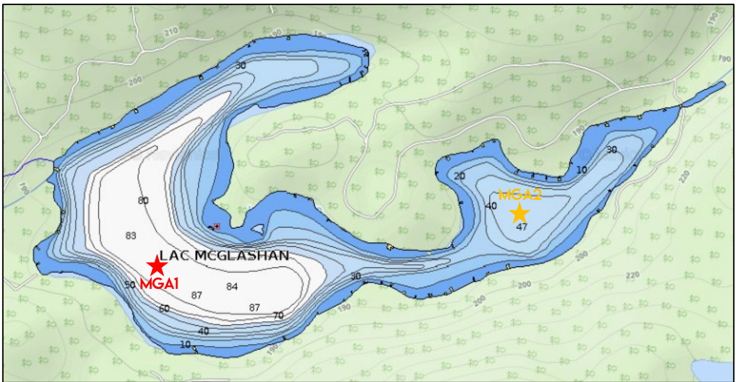
Figure 5 – Carte bathymétrique du lac McGlashan (Navionics, 2021)
