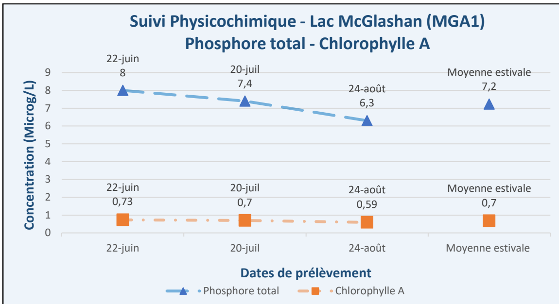
Figure 7 – Résultats – Suivi physicochimique 2025 (PT, Chla) – Lac McGlashan (MGA1)
