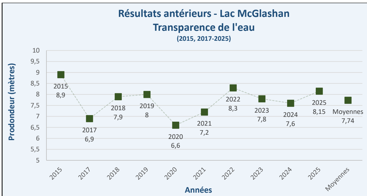
Figure 11 – Résultats antérieurs – Transparence de l'eau – Lac McGlashan
