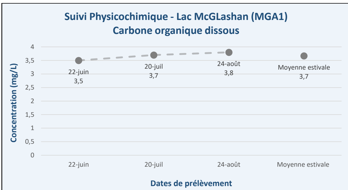
Figure 8 – Résultats – Suivi physicochimique 2025 (COD) – Lac McGlashan (MGA1)
