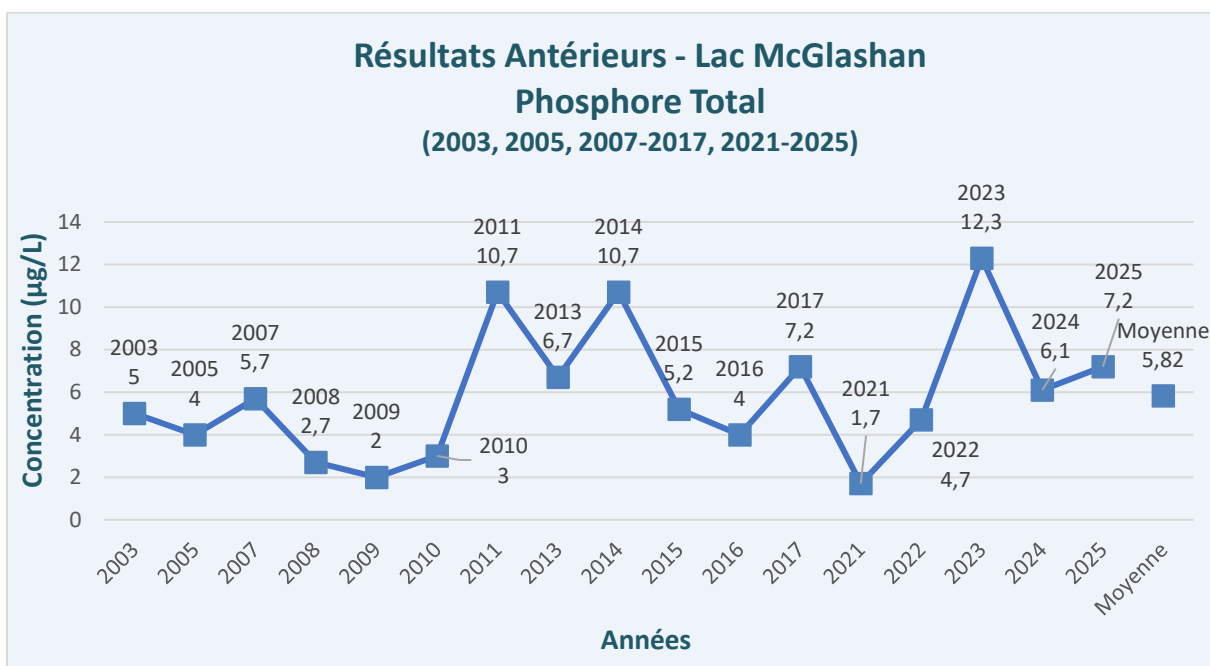
Figure 10 – Résultats antérieurs – Phosphore total – Lac McGlashan
