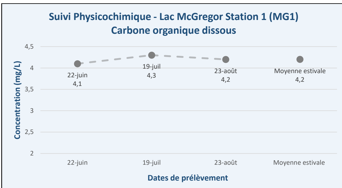
Figure 7 – Résultats – Suivi physicochimique 2025 (COD) – Lac McGregor (MG1)
