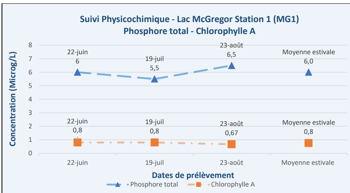
Figure 6 – Résultats – Suivi physicochimique 2025 (PT, Chla) – Lac McGregor (MG1)
