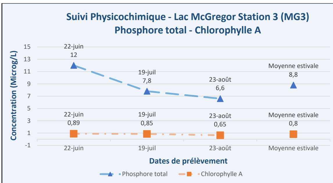
Figure 10 – Résultats – Suivi physicochimique 2025 (PT, Chla) – Lac McGregor (MG3)
