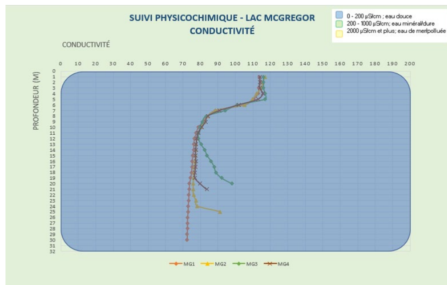
Figure 12 – Résultats – Profils physicochimiques 2024 – Lac McGregor
