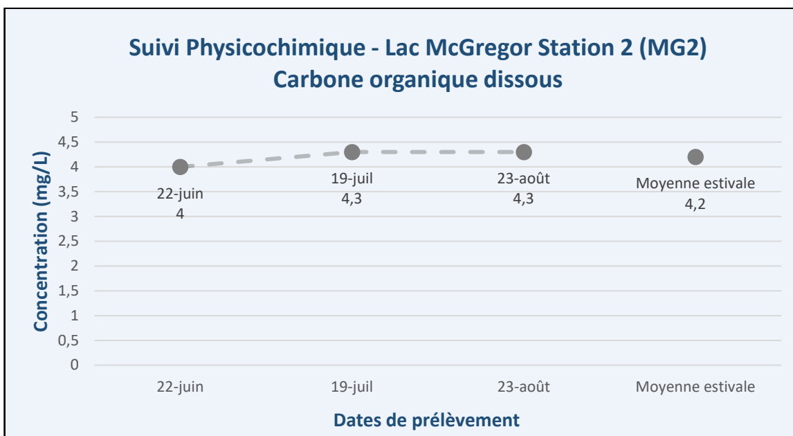
Figure 9 – Résultats – Suivi physicochimique 2025 (COD) – Lac McGregor (MG2)
