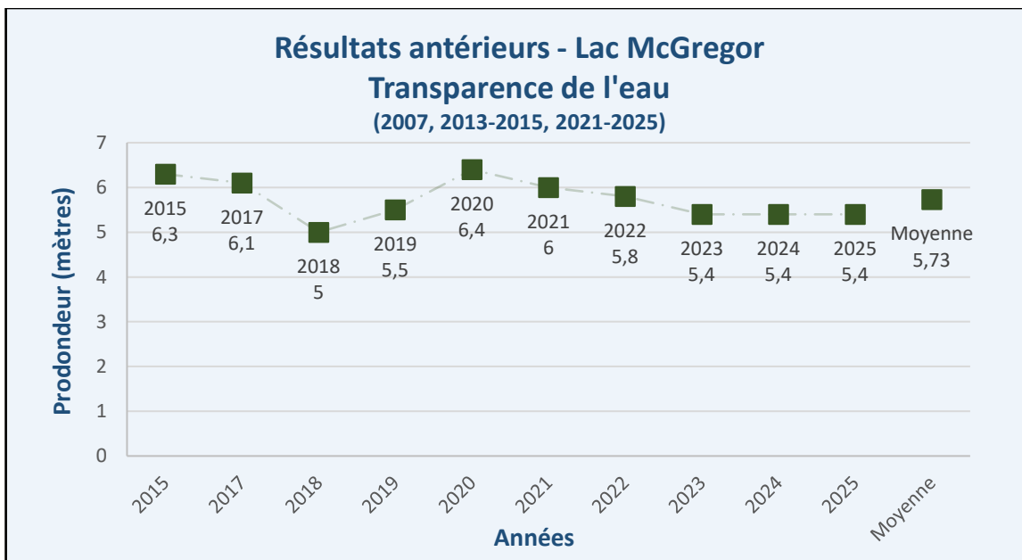
Figure 13 – Résultats antérieurs – Transparence de l'eau – Lac McGregor
