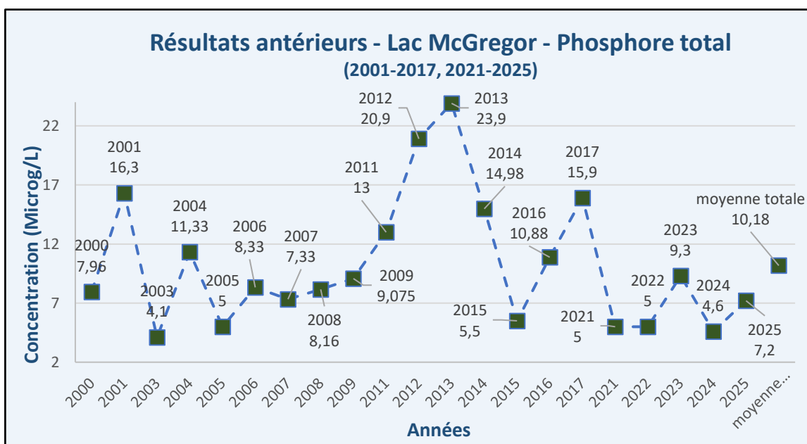
Figure 14 – Résultats antérieurs – Phosphore total – Lac McGregor
