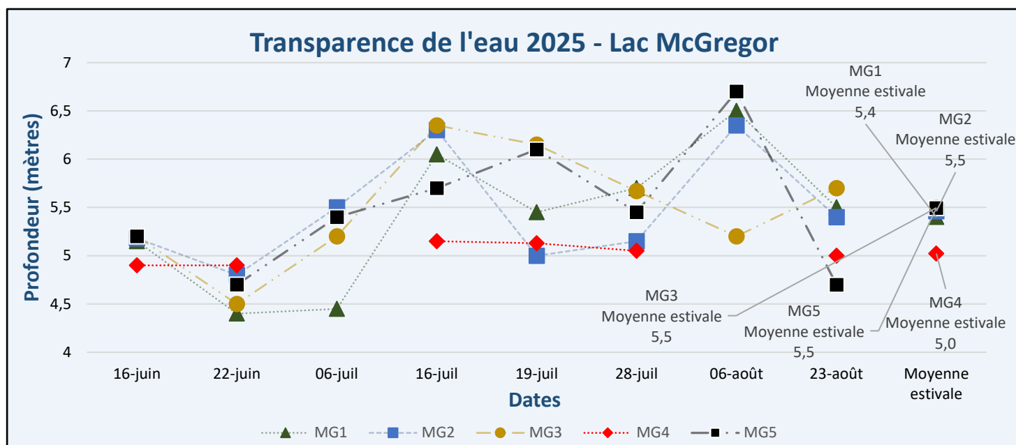
Figure 5 – Résultats – Transparence de l'eau 2025 – Lac McGregor
