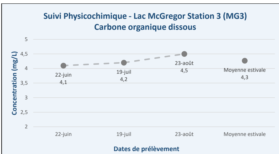
Figure 11 – Résultats – Suivi physicochimique 2025 (COD) – Lac McGregor (MG3)
