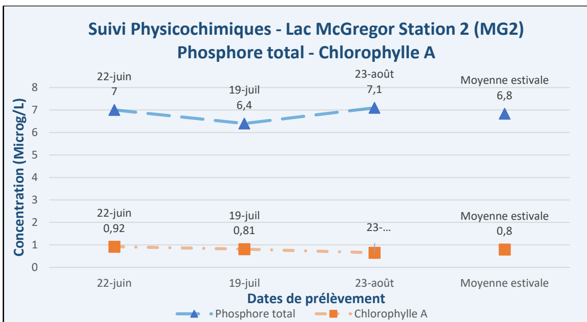
Figure 8 – Résultats – Suivi physicochimique 2025 (PT, Chla) – Lac McGregor (MG2)
