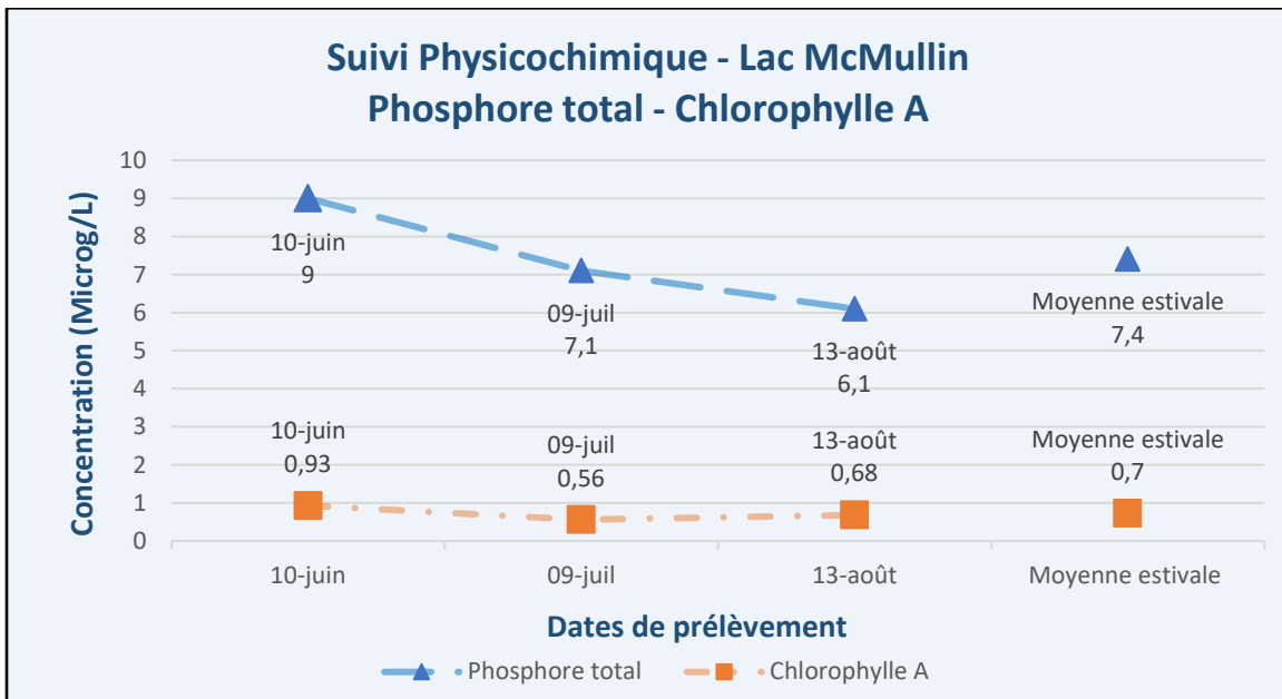
Figure 6 – Résultats – Suivi physicochimique 2025 (PT, Chla) – Lac McMullin (MU1)
