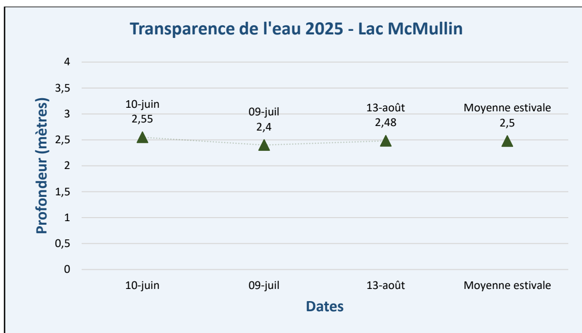
Figure 5 – Résultats – Transparence de l'eau 2025 – Lac McMullin
