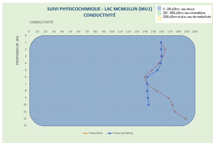
Figure 8 – Résultats – Profils physicochimiques 2024 – Lac McMullin (MU1)
