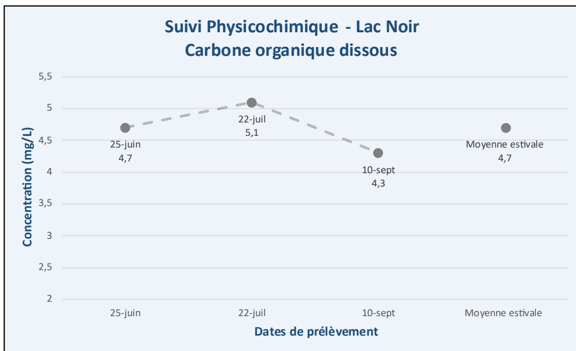
Figure 8 – Résultats – Suivi physicochimique 2024 (COD) – Lac Noir (N1)
