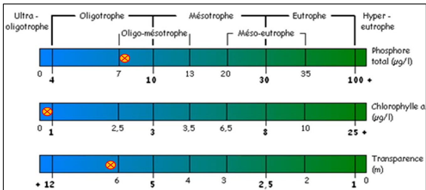
Figure 10 – État trophique 2024 – Lac Noir (N1)
