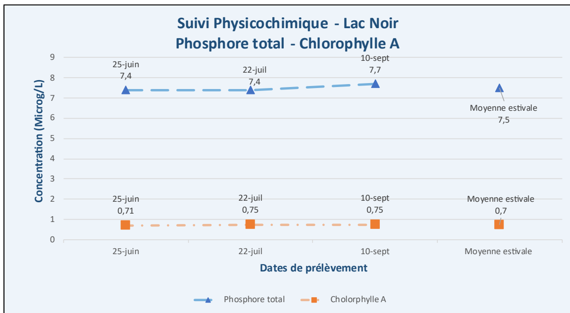
Figure 7 – Résultats – Suivi physicochimique 2025 (PT, Chla) – Lac Noir (N1)
