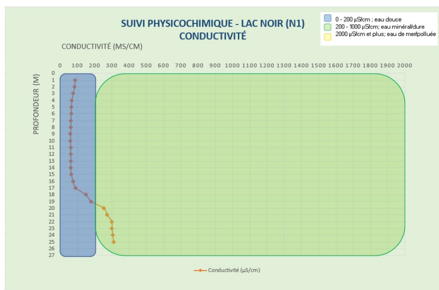
Figure 9 – Résultats – Profils physicochimiques 2024 – Lac Noir (N1)
