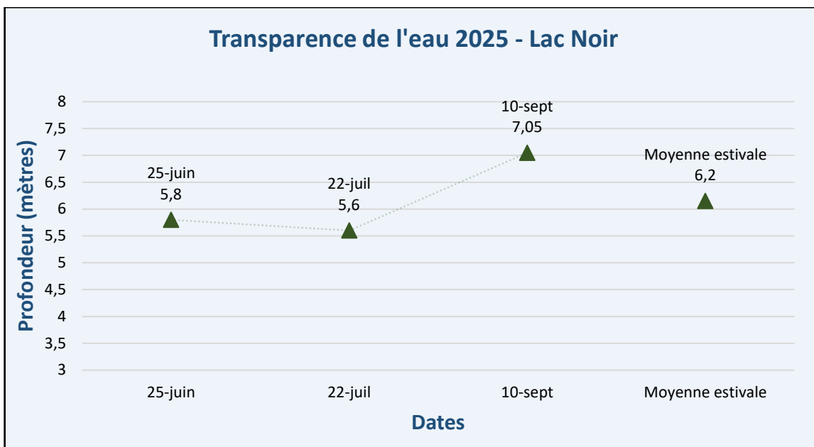
Figure 6 – Résultats – Transparence de l'eau 2025 – Lac Noir
