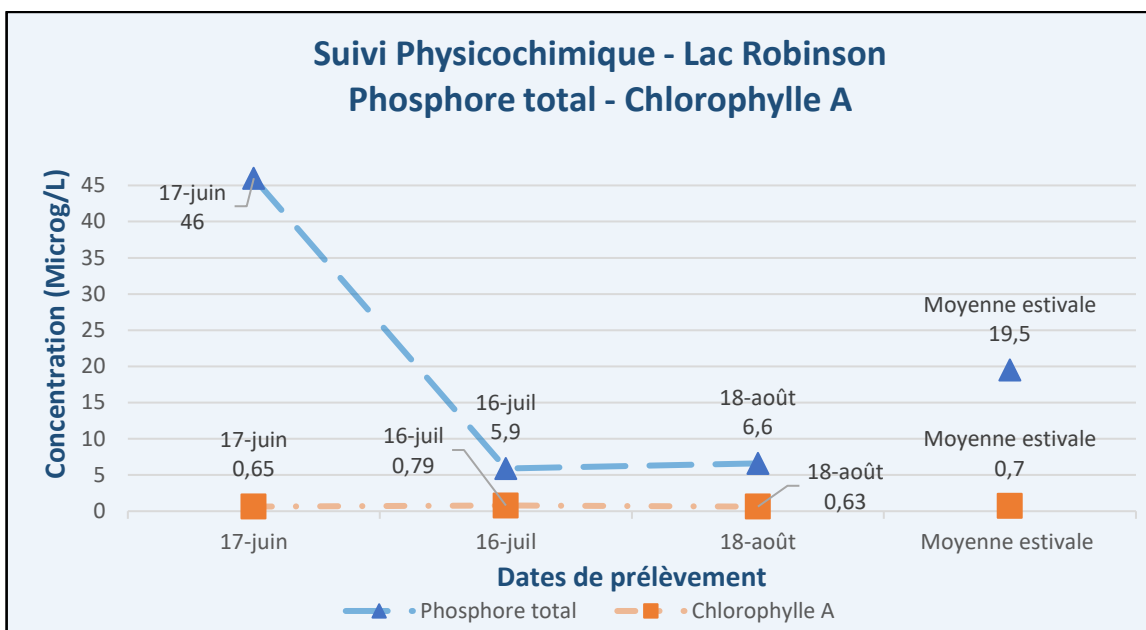
Figure 6 – Résultats – Suivi physicochimique 2025 (PT, Chla) – Lac Robinson (Rob1)
