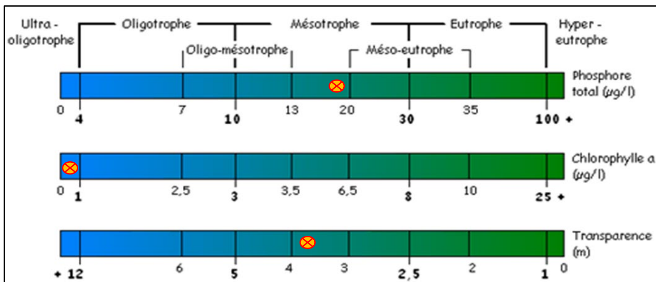
Figure 9 – État trophique 2025 – Station 1 – Lac Robinson (Rob1)
