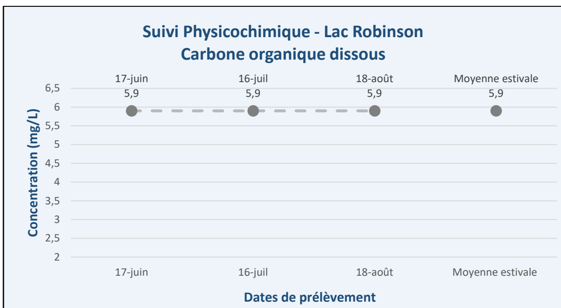
Figure 7 – Résultats – Suivi physicochimique 2025 (COD) – Lac Robinson (Rob1)
