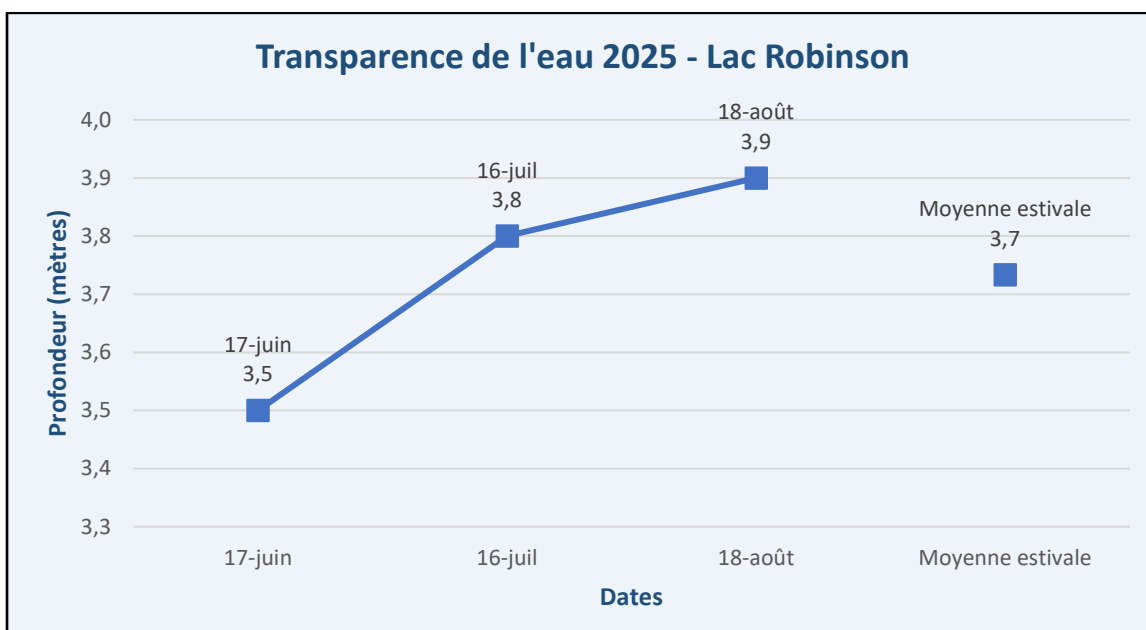
Figure 5 – Résultats – Transparence de l'eau 2025 – Lac Robinson (Rob1)
