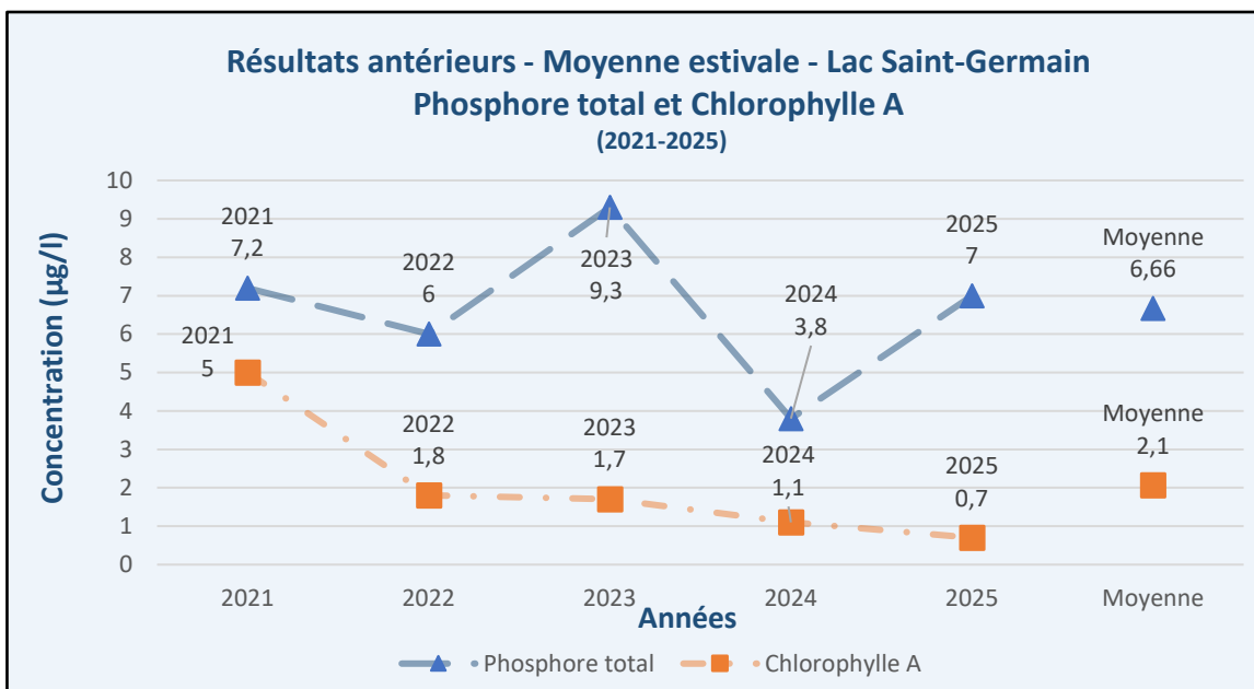
Figure 13 - Résultats antérieurs – Phosphore total – Chlorophylle A – Lac Saint-Germain
