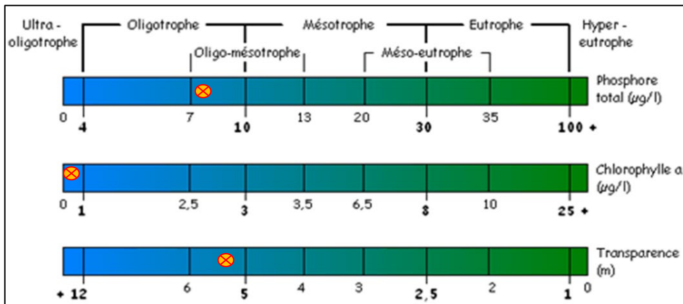
Figure 15 – État trophique 2025 – Station 1 – Lac Saint-Germain (SG1)
