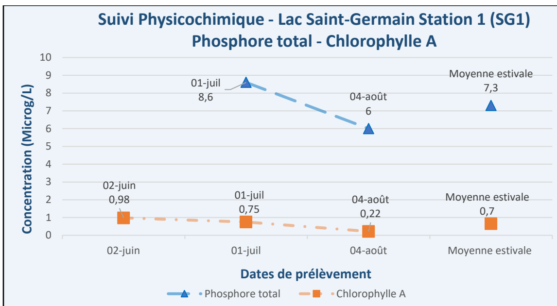
Figure 6 – Résultats – Suivi physicochimique 2025 (PT, Chla) – Lac Saint-Germain (SG1)
