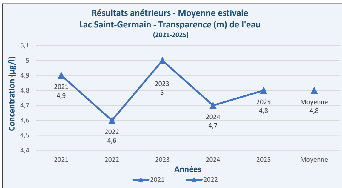
Figure 14 – Résultats antérieurs – Transparence (m) de l'eau 2025 - Lac Saint-Germain
