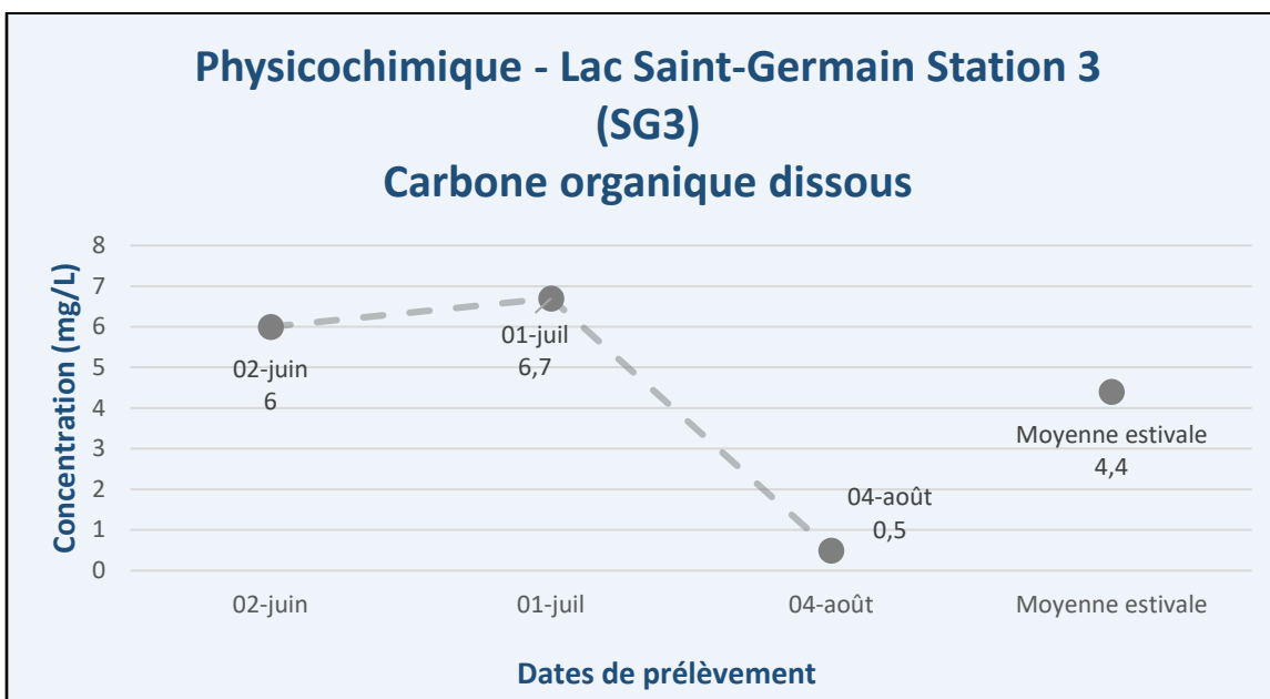
Figure 11 – Résultats – Suivi physicochimique 2025 (COD) – Lac Saint-Germain (SG3)
