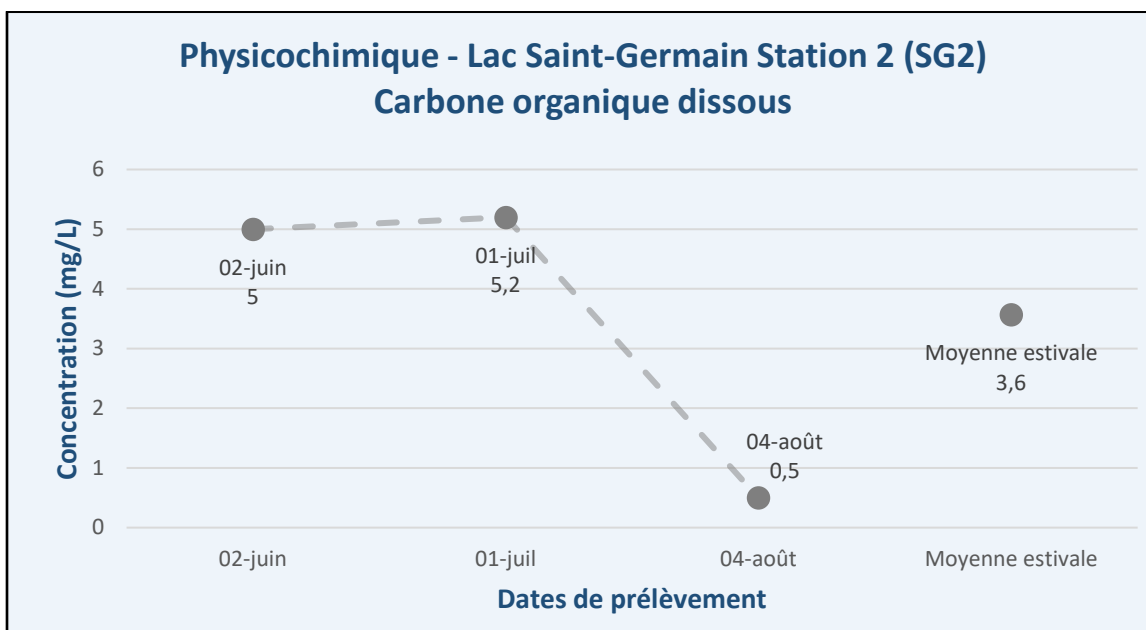
Figure 9 – Résultats – Suivi physicochimique 2025 (COD) – Lac Saint-Germain (SG2)
