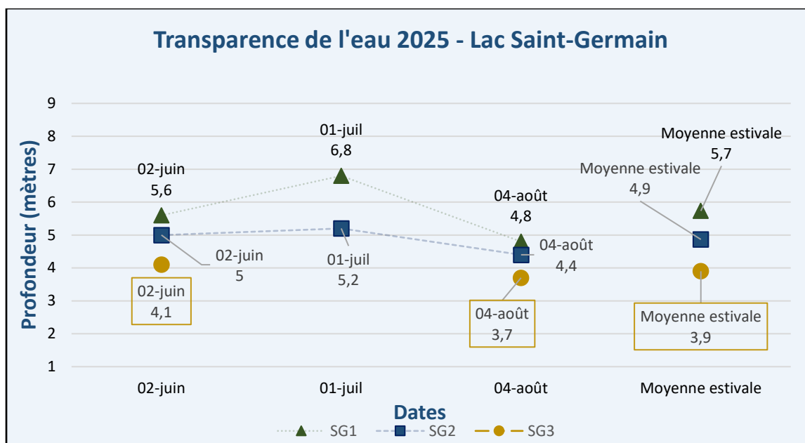
Figure 5 – Résultats – Transparence de l'eau 2025 - Lac Saint-Germain
