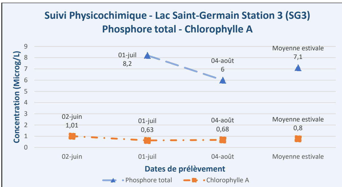
Figure 10 – Résultats – Suivi physicochimique 2025 (PT,Chla) – Lac Saint-Germain (SG3)
