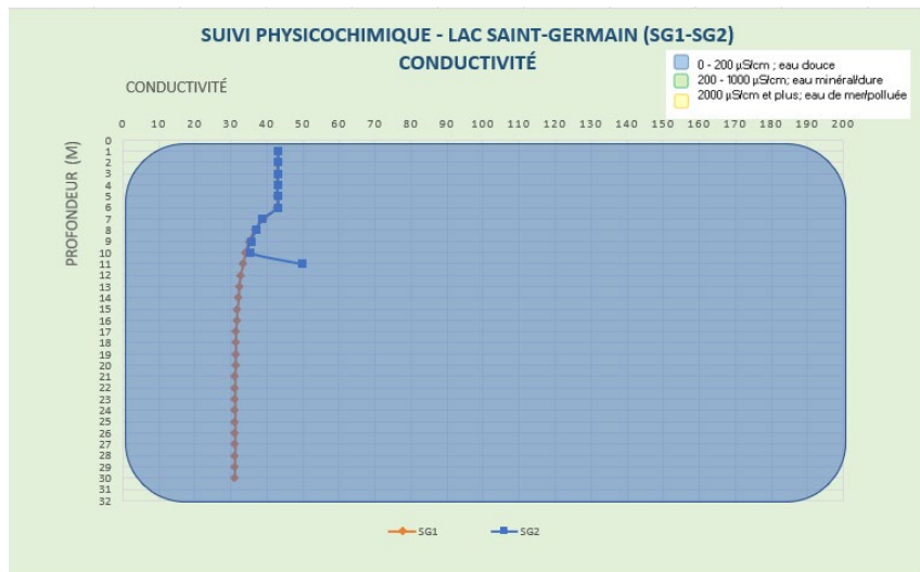
Figure 12 – Résultats – Profils physicochimiques 2024 – Lac Saint-Germain (SG1) – (SG2)
