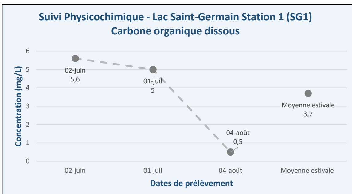
Figure 7 – Résultats – Suivi physicochimique 2025 (COD) – Lac Saint-Germain (SG1)
