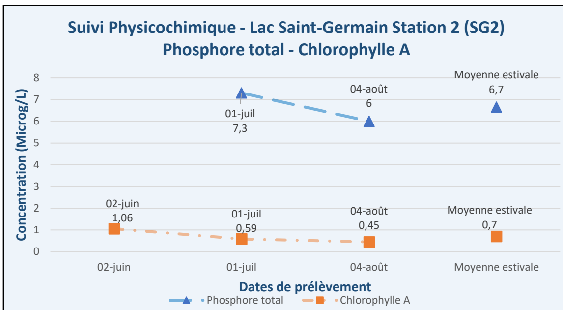
Figure 8 – Résultats – Suivi physicochimique 2025 (PT, Chla) – Lac Saint-Germain (SG2)
