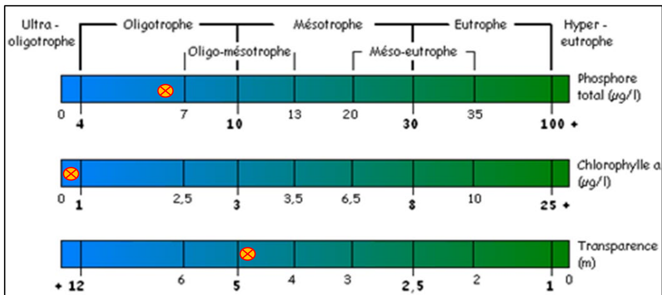
Figure 16 – État trophique 2025 – Station 2 – Lac Saint-Germain (SG2)
