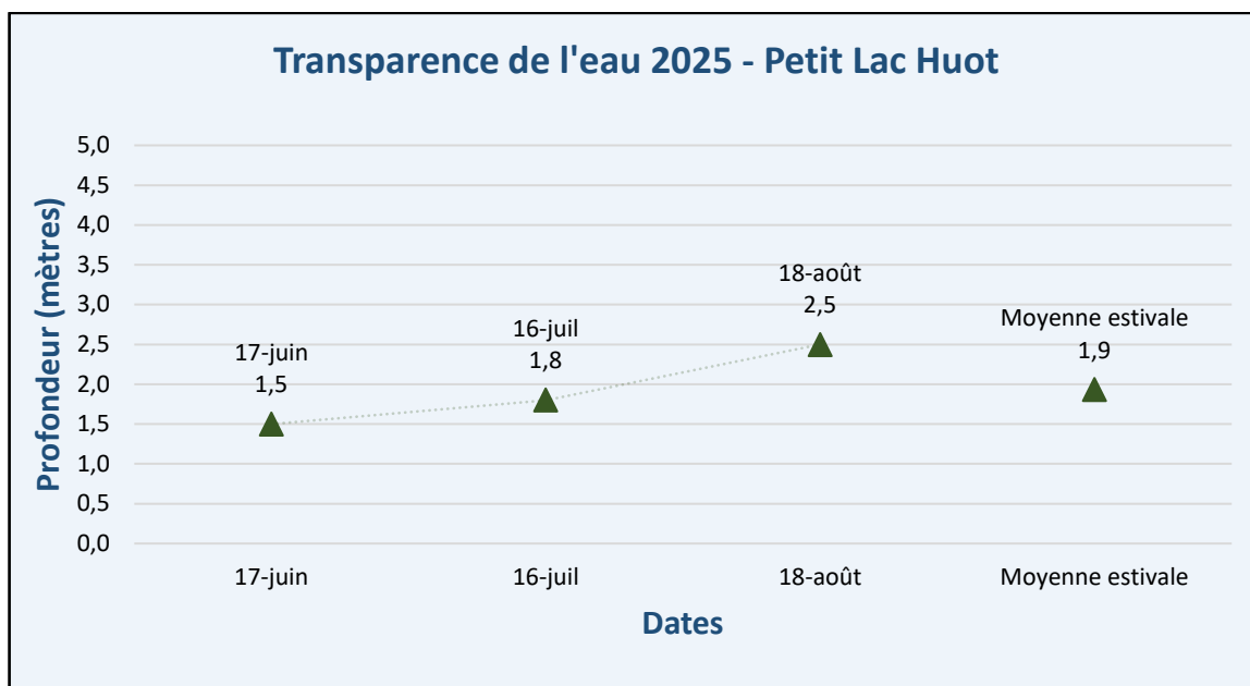
Figure 6 – Résultats – Transparence de l'eau 2025 – Petit lac Huot
