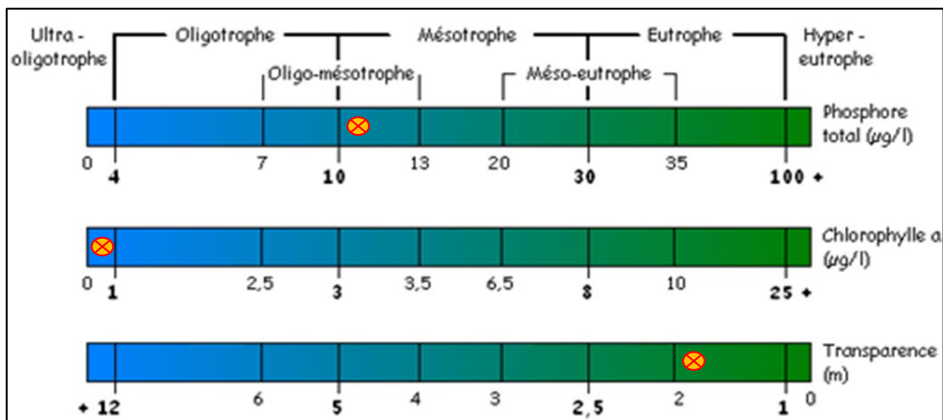
Figure 10 – État trophique 2025 – Petit Lac Huot (PLH1)
