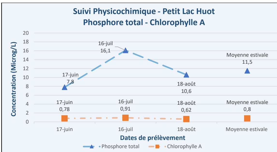
Figure 7 – Résultats – Suivi physicochimique 2025 (PT, Chla) – Petit Lac Huot (PLH1)
