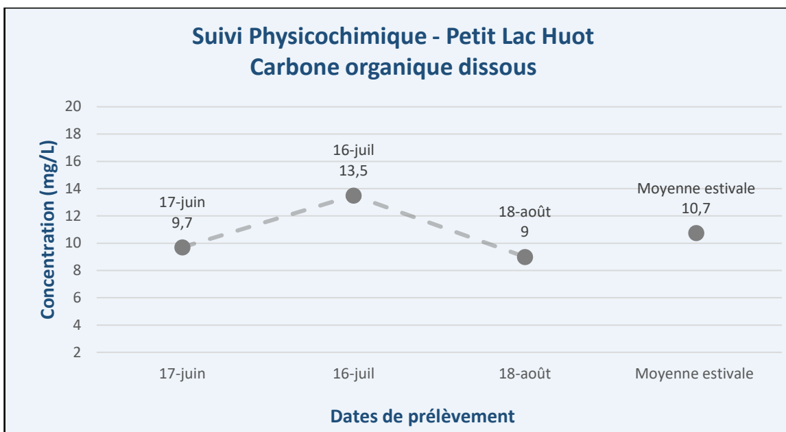
Figure 8 – Résultats – Suivi physicochimique 2025 (COD) – Petit lac huot (PLH1)
